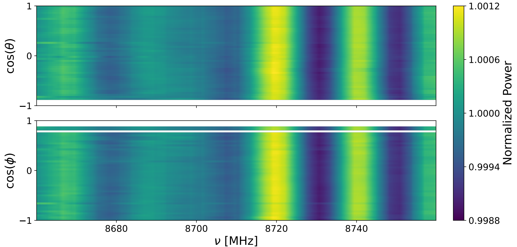
Bank 1 decay: 8660-8760 MHz
