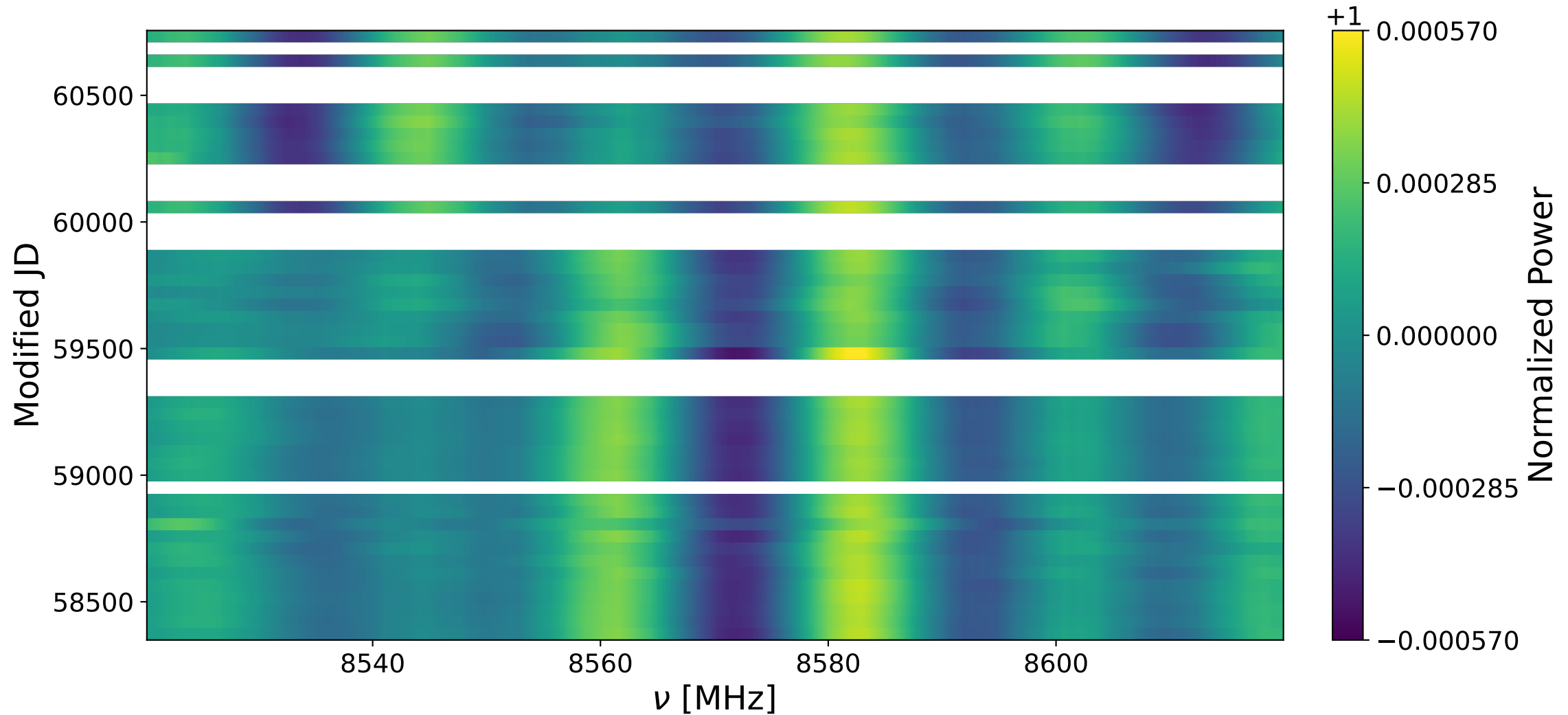
Bank 0 decay: 8520-8620 MHz
