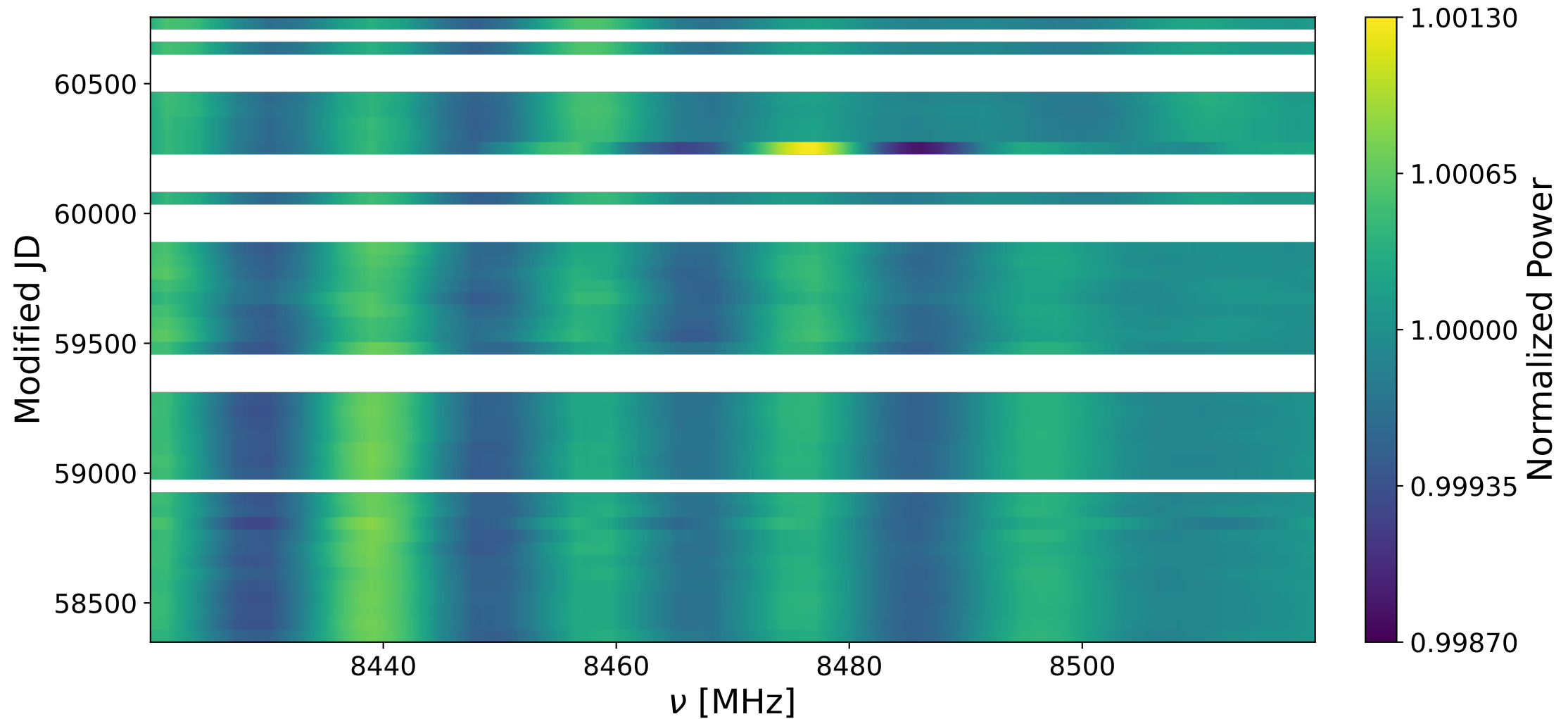
Bank 0 decay: 8420-8520 MHz
