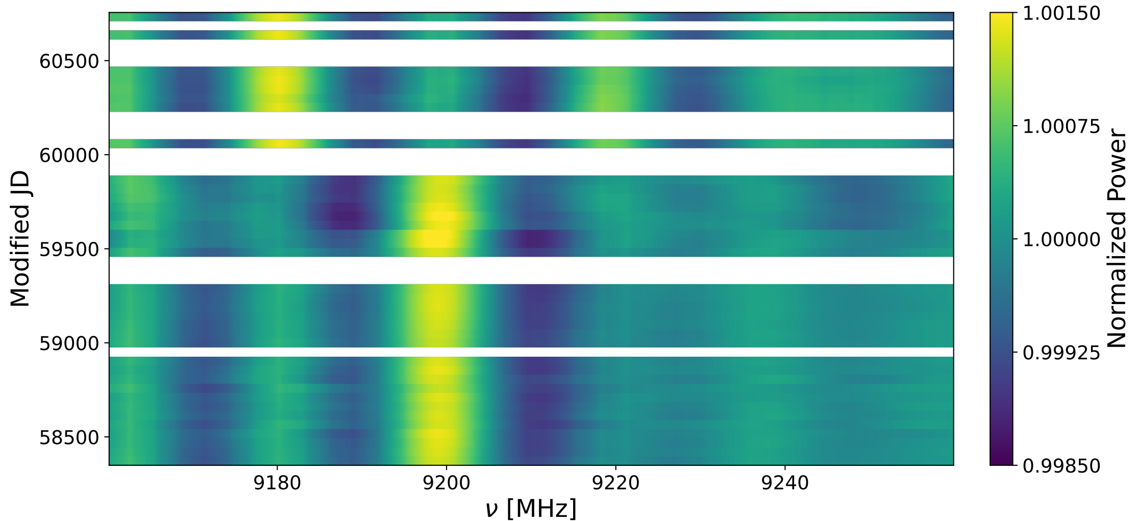
Bank 1 decay: 9160-9260 MHz
