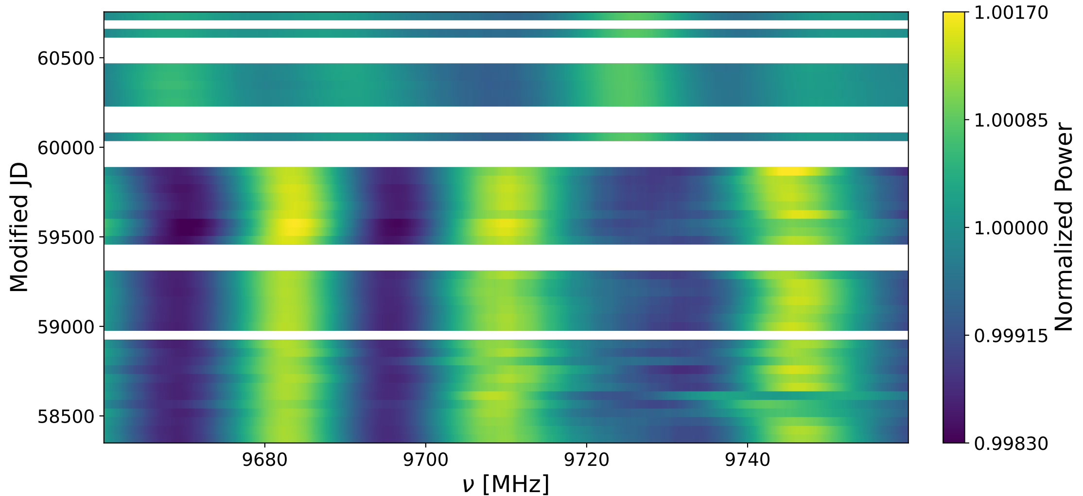
Bank 1 decay: 9660-9760 MHz
