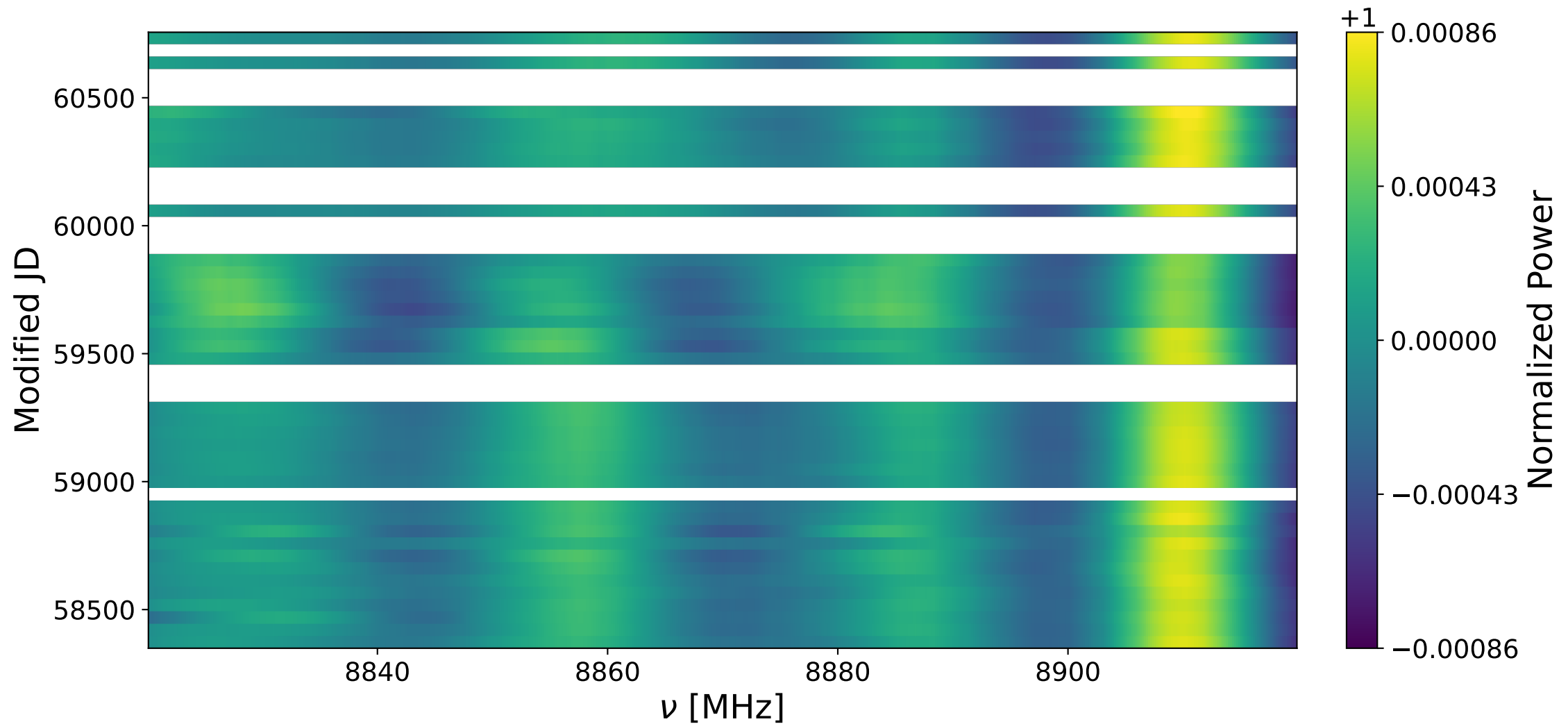
Bank 0 decay: 8820-8920 MHz
