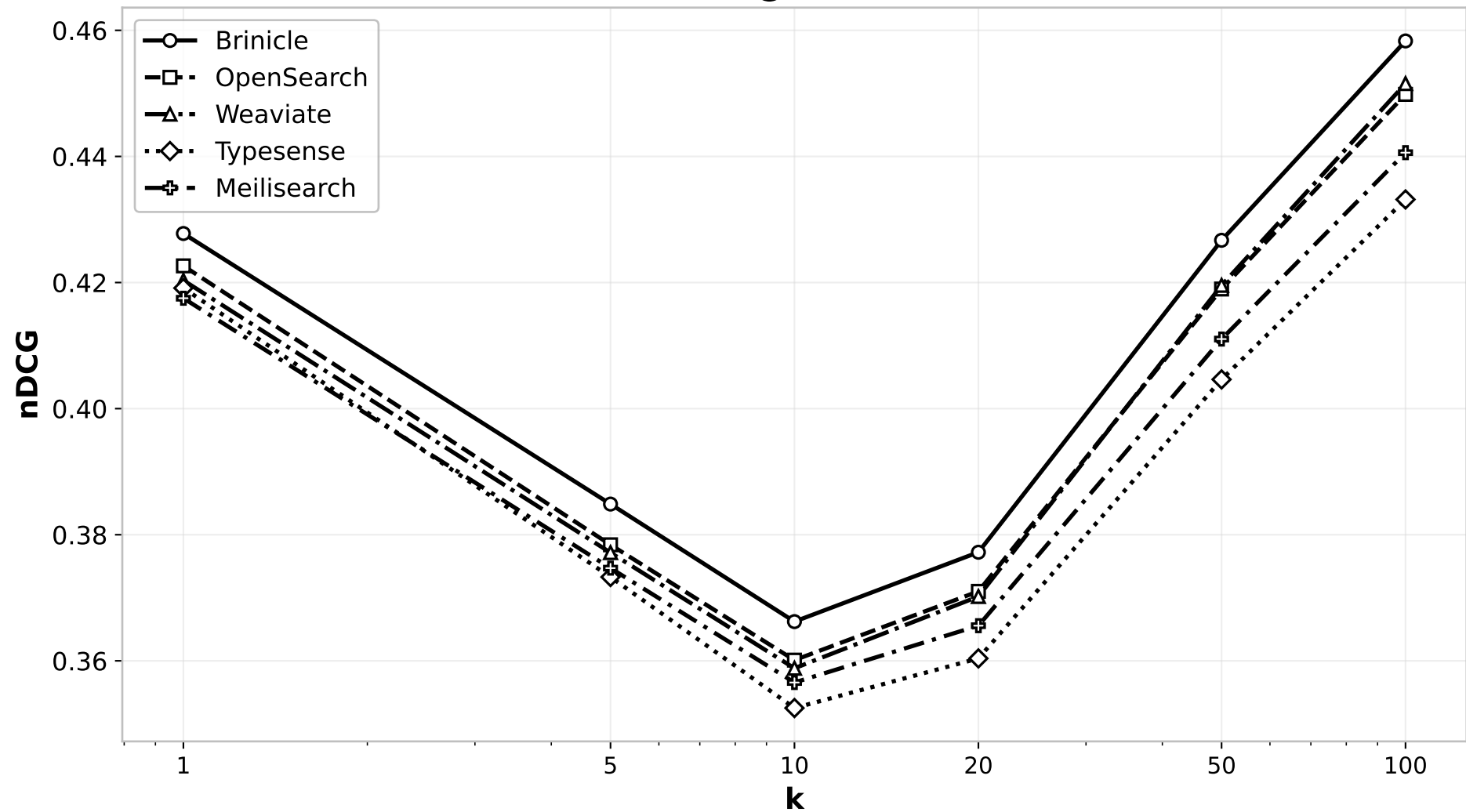
nDCG@k (ESCI)
