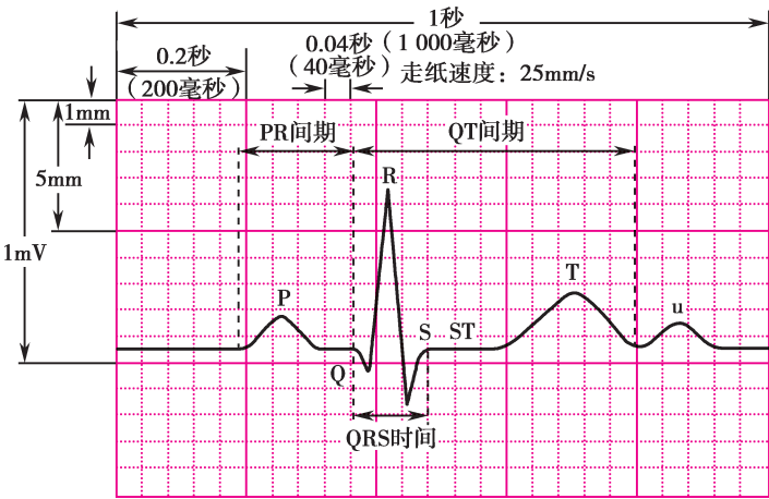
图 5-1-13 心电图各波段的测量
