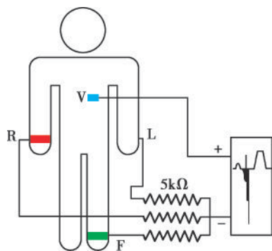
图 5-1-11 胸导联电极的连接方式
