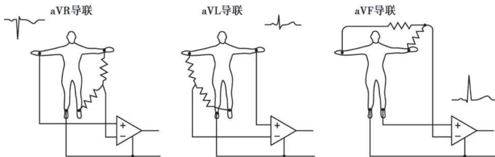
图 5-1-10 加压肢体导联的电极位置及电极连接方式
