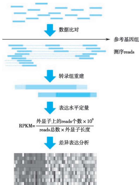
图 16-2 RNA-seq 测序数据分析流程示意图
