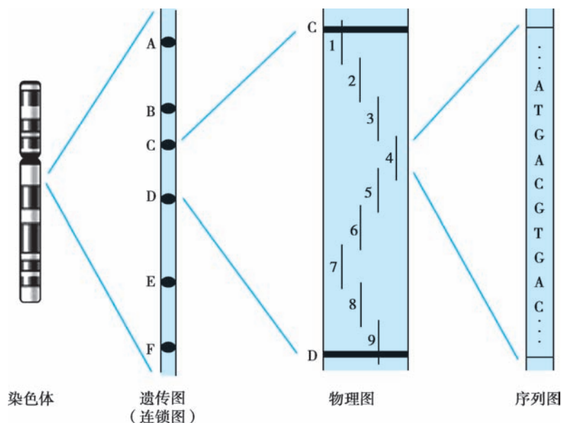
图 14-1 人类基因组计划主要目标图解
