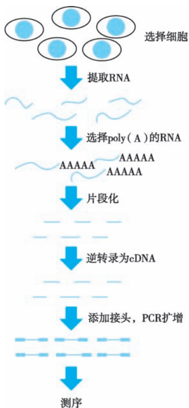
图 16-1 RNA-seq 测序流程示意图
