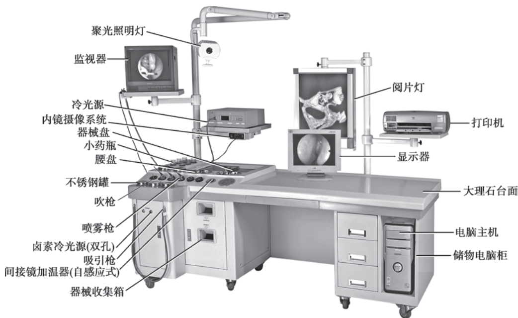
图 1-2-5 耳鼻咽喉头颈外科诊查综合治疗工作台
