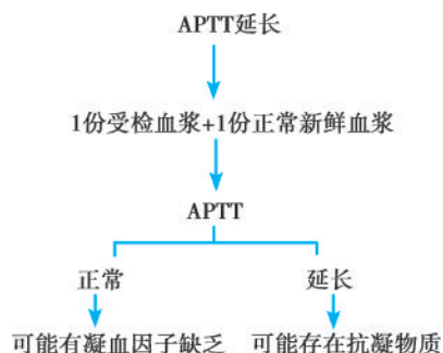
图 4-3-2 APTT 延长混合血浆纠正试验
