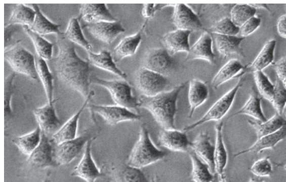
图 1-8 HeLa 细胞相差显微镜图
