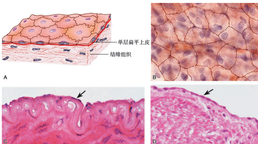
图 2-1 单层扁平上皮
