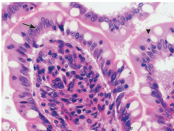
图 1-1 HE 染色的小肠绒毛光镜图
