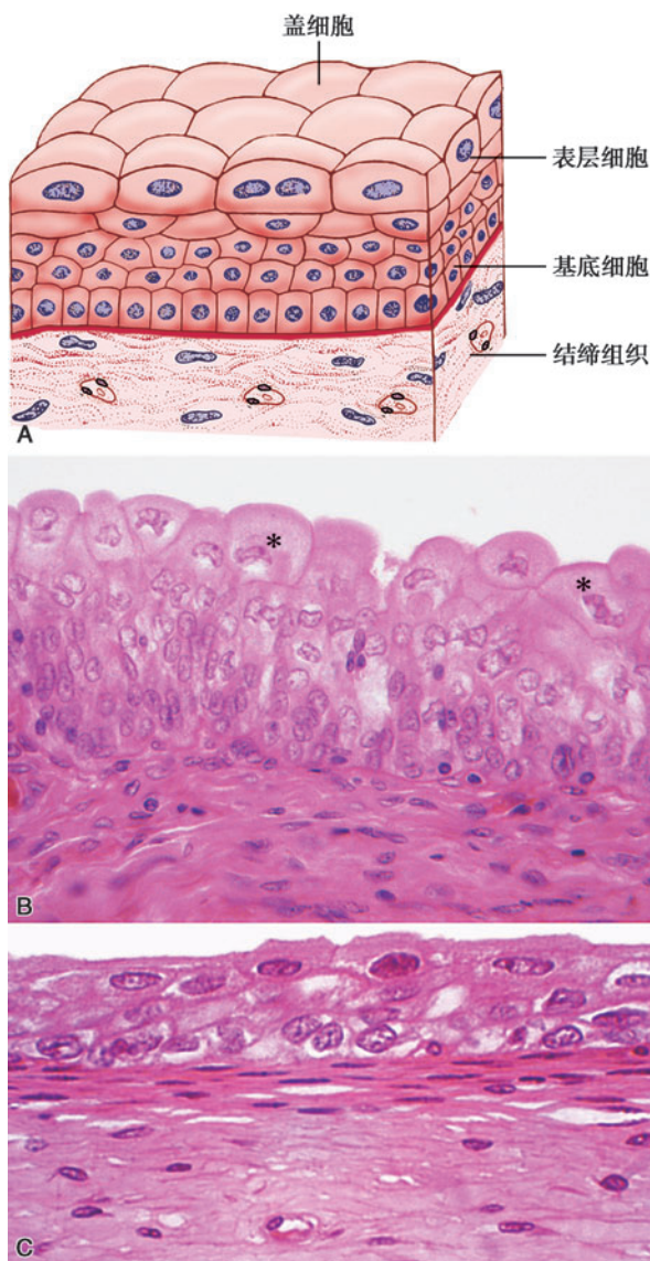
图 2-7 变移上皮
