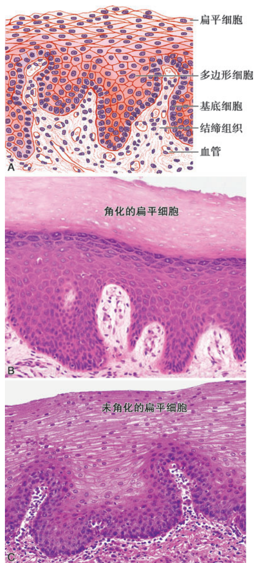
图 2-6 复层扁平上皮
