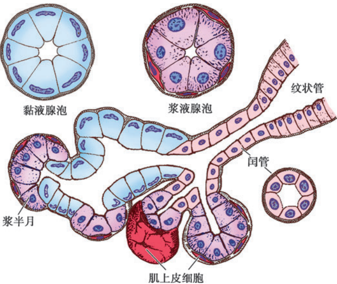
图 2-9 外分泌腺结构与腺泡类型模式图
