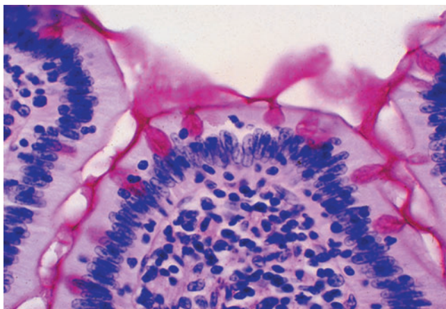
图 1-2 小肠光镜图
