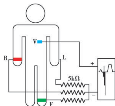
图 5-1-11 胸导联电极的连接方式
