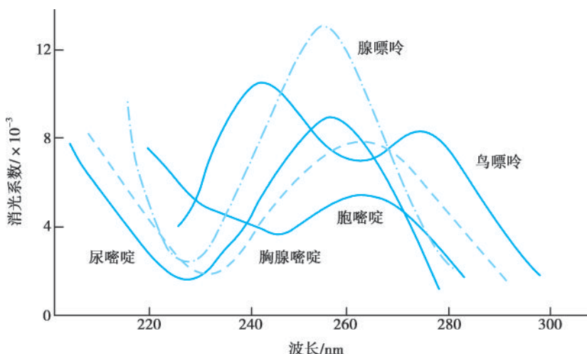
图 3-26 五种碱基的紫外吸收光谱 (pH 7.0)
