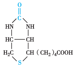
图 6-8 生物素的结构
