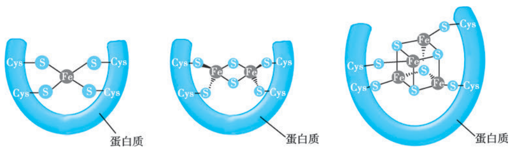
图 10-7 铁硫中心的结构 S表示无机硫。
