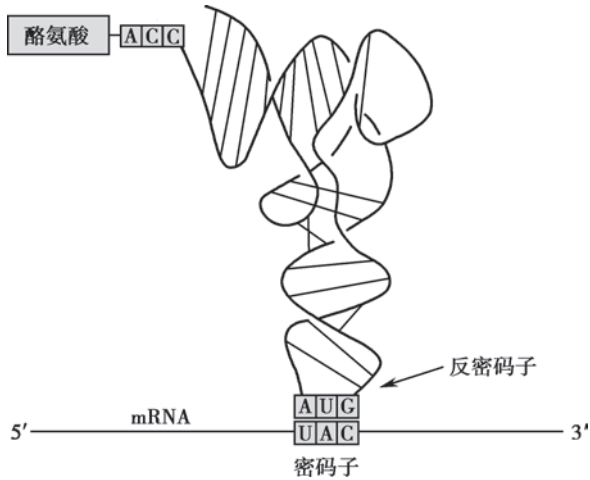
图 3-23 tRNA 反密码子与 mRNA 密码子相互识别的示意图 在蛋白质生物合成过程中,通过正确的碱基配对,mRNA 密码子与密码子所编码的氨基酸建立了一一对应的关系。
