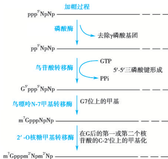
图 15-13 真核 mRNA 的 5'-帽结构及加帽过程
