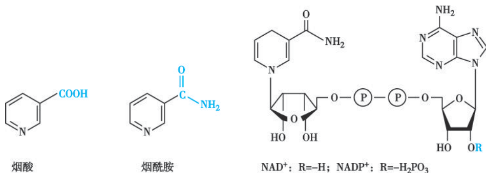
图 6-6 维生素 PP 及其活性形式的结构
