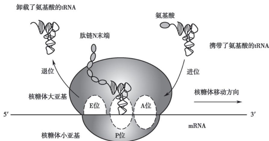
图 3-25 由核糖体、mRNA 和 tRNA 形成的复合体
