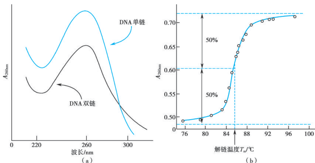
图 3-28 DNA 解链过程中的增色效应和对应的解链曲线
