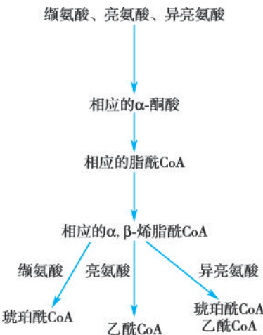
图 9-13 支链氨基酸的分解代谢
