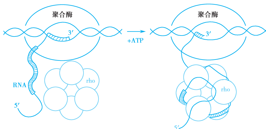
图 15-7 依赖 \rho 因子的转录终止
