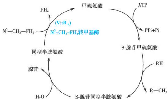
图 9-11 甲硫氨酸循环
