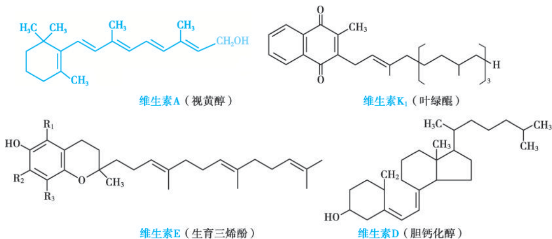
图 6-1 脂溶维生素的结构
