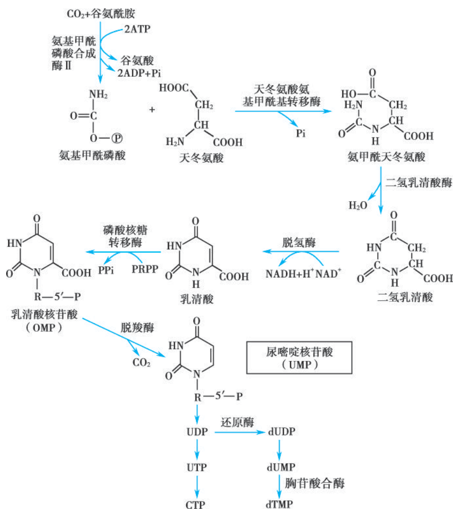
图 11-11 嘧啶核苷酸的合成代谢
