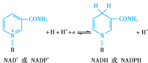
图 10-4 NAD(P) + 的加氢和 NAD(P)H 的脱氢反应
