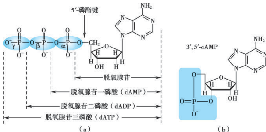
图 3-5 核苷酸的化学结构
