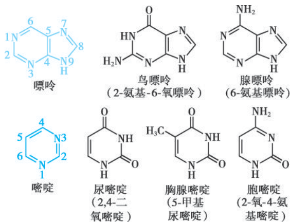
图 3-1 构成核苷酸的嘌呤和嘧啶的化学结构式
