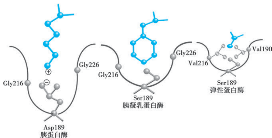
图 2-9 胰蛋白酶、胰凝乳蛋白酶和弹性蛋白酶与底物结合时的“口袋”状活性中心
