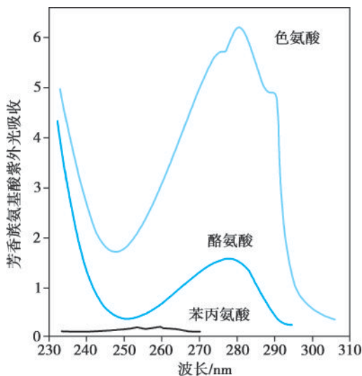
图 1-3 芳香族氨基酸的紫外线吸收对比
