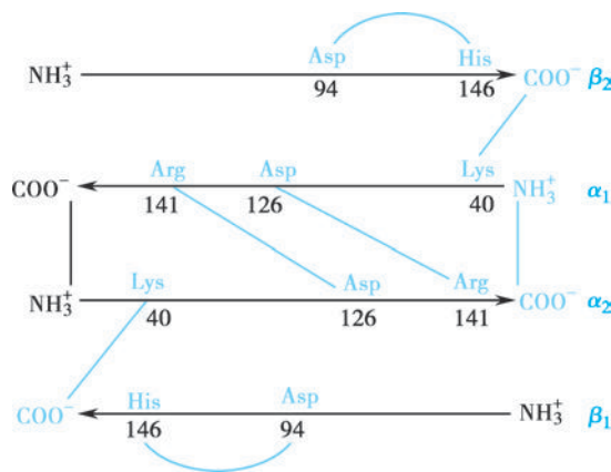
图 1-25 脱氧 Hb 亚基间和亚基内的盐键
