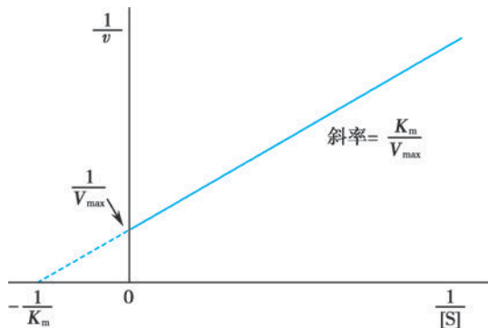
图 2-12 双倒数作图法
