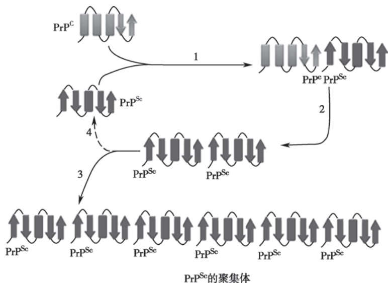
图 1-30 PrP C 转变成 PrP Sc 的过程
