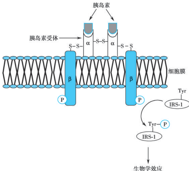
图 1-18 胰岛素与胰岛素受体结合,启动胰岛素信号通路
