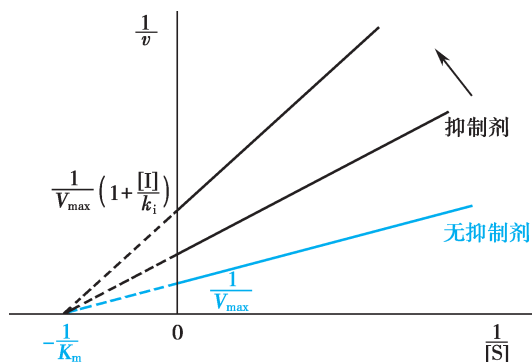
图 2-18 非竞争性抑制双倒数作图
