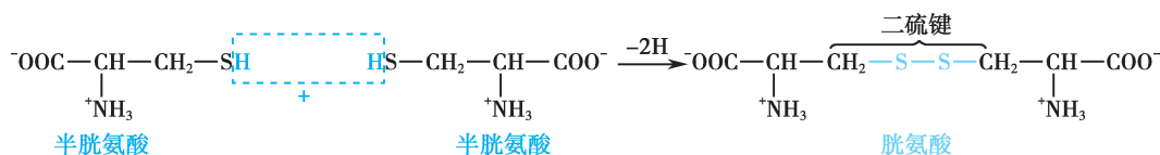
图 1-2 胱氨酸和二硫键
