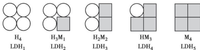
图 2-3 乳酸脱氢酶同工酶的亚基构成
