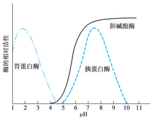
图 2-15 pH 对胃蛋白酶、胆碱酯酶和胰蛋白酶活性的影响
