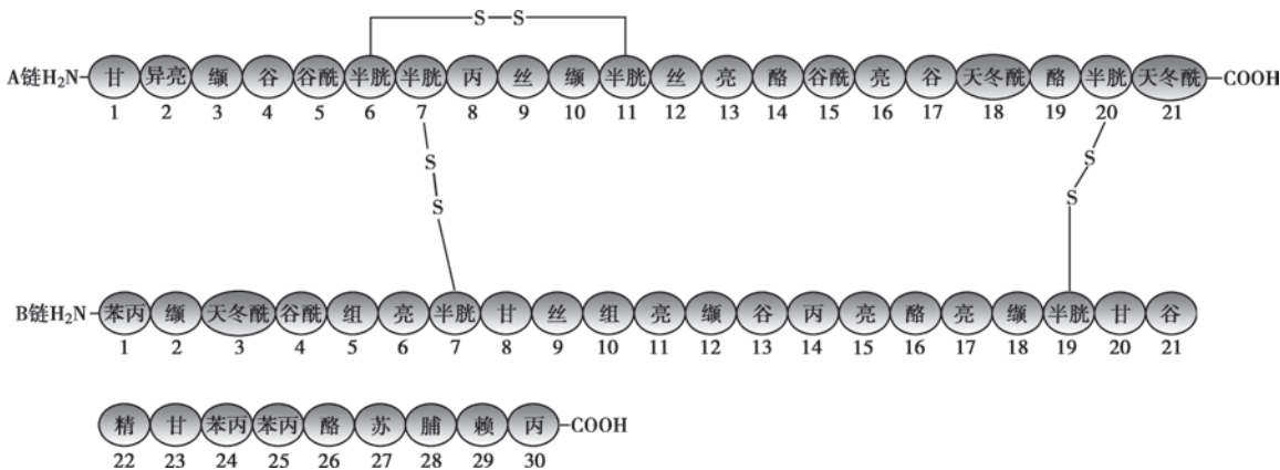
图 1-8 牛胰岛素的一级结构
