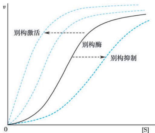
图 2-20 别构酶的正协同效应速率-底物浓度作图 别构激活剂使别构酶的 S 形曲线左移,别构抑制剂使 S 形曲线右移。
