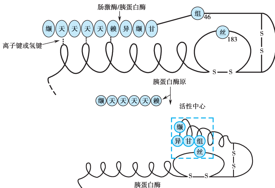
图 2-22 胰蛋白酶原的激活示意图
