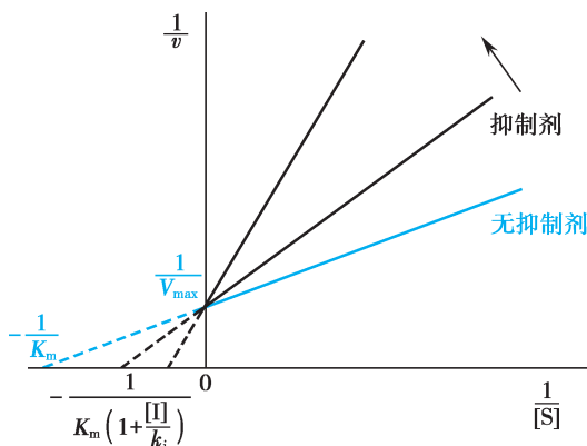
图 2-16 竞争性抑制双倒数作图
