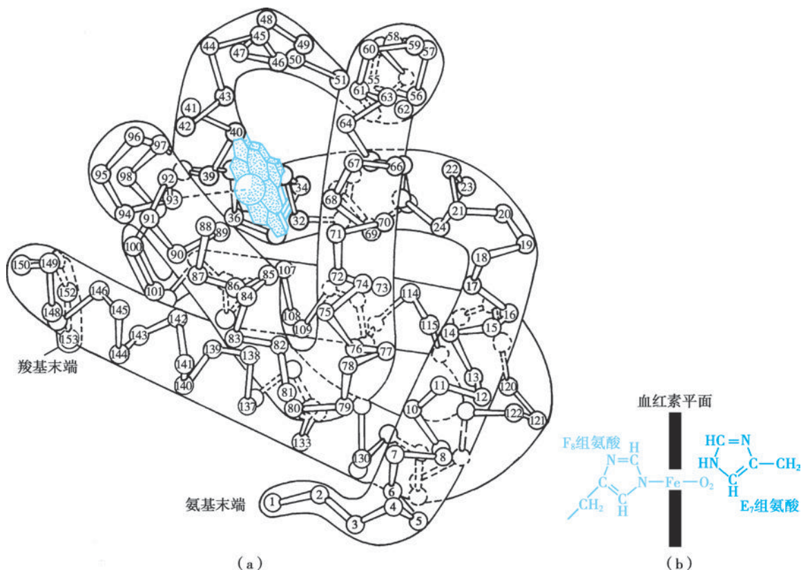
图 1-13 肌红蛋白中血红素与肽链的关系
