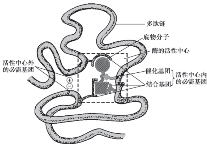
图 2-1 酶的活性中心示意图
