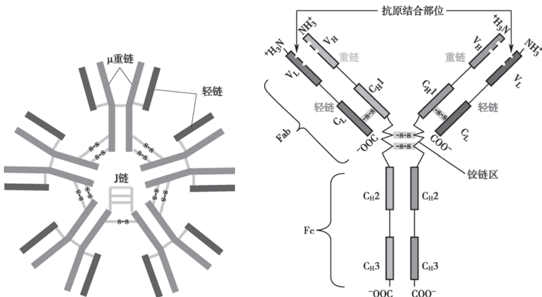
图 1-19 IgM 的五聚体形式
