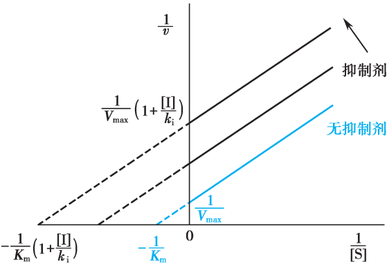
图 2-19 反竞争性抑制双倒数作图
