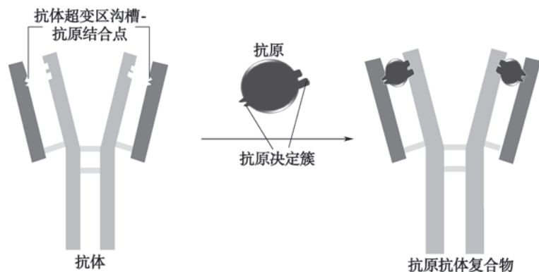
图 1-21 抗原 - 抗体的特异性结合
