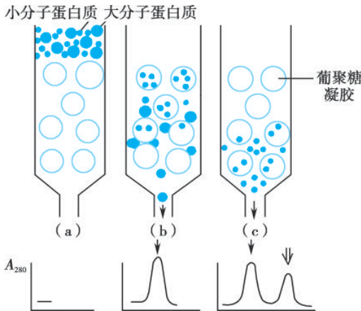
图 1-32 凝胶过滤分离蛋白质 (a) 大球是葡聚糖凝胶颗粒;(b) 样品上柱后,小分子进入凝胶微孔,大分子不能进入,故洗脱时大分子先洗脱下来;(c) 小分子后洗脱出来。
