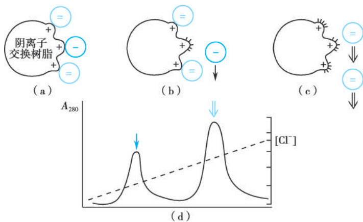
图 1-31 离子交换层析分离蛋白质 (a) 样品全部交换并吸附到树脂上;(b) 负电荷较少的分子用较稀的 Cl - 或其他负离子溶液洗脱;(c) 电荷多的分子随 Cl - 浓度增加依次洗脱;(d) 洗脱图 A 280 表示为 280nm 的吸光度。
