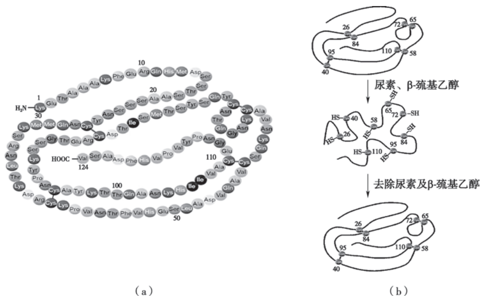
图 1-22 牛核糖核酸酶 A 一级结构与空间结构的关系
