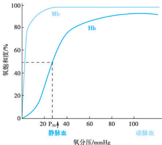
图 1-26 Hb 和 Mb 的氧解离曲线
