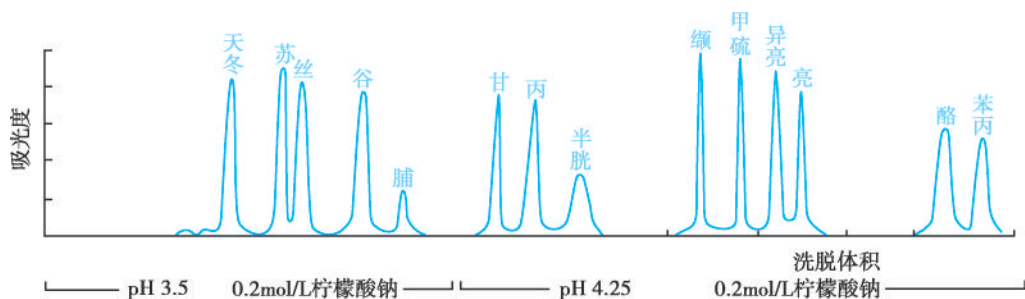
图 1-33 离子交换层析分析蛋白质的氨基酸组分
