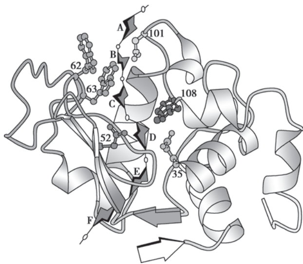
图 2-2 溶菌酶的活性中心
