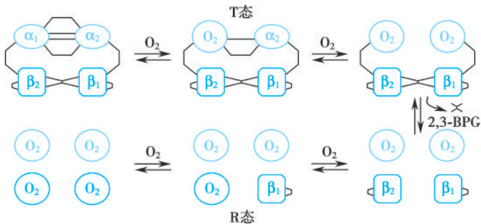
图 1-28 Hb 氧合与脱氧构象转换示意
