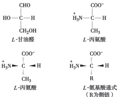
图 1-1 L-甘油醛和 L-氨基酸
