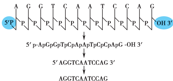
图 3-7 核酸的一级结构以及书写法
