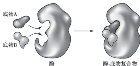
图 2-8 酶与底物的邻近效应与定向排列
