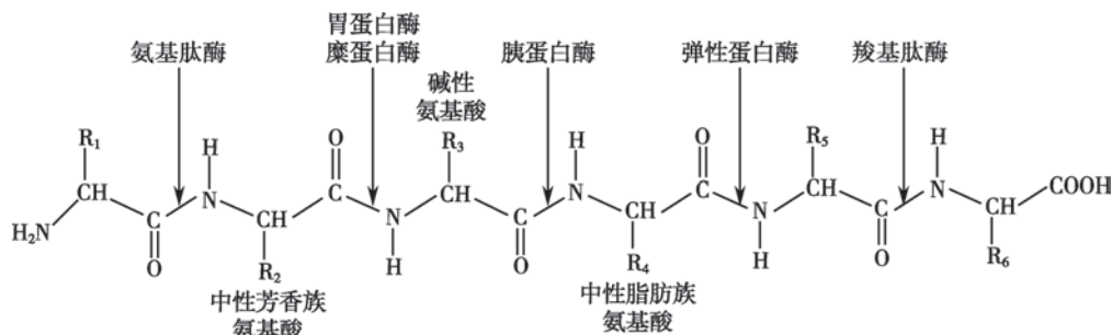
图 2-5 消化道中各种蛋白酶对肽键的专一性
