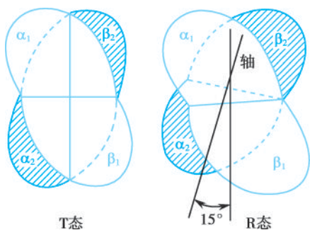
图 1-27 Hb T 态和 R 态互变
