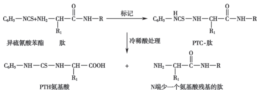
图 1-34 肽的氨基酸末端测定法
