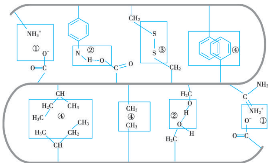
图 1-14 维持蛋白质分子构象的各种化学键
