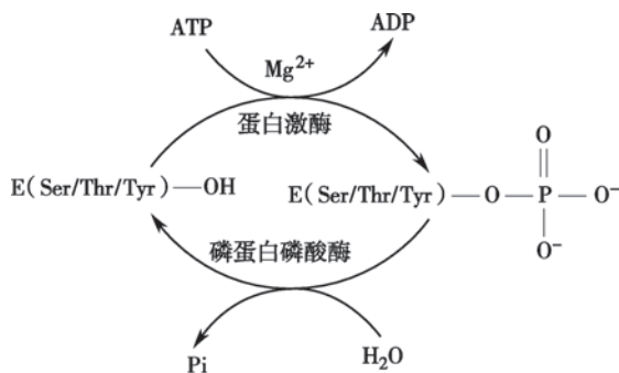
图 2-21 酶的磷酸化和去磷酸化调节
