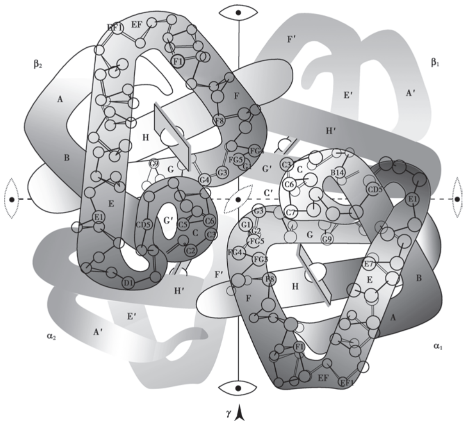
图 1-17 蛋白质的四级结构——血红蛋白结构示意图
