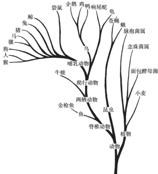
图 1-23 细胞色素 c 的生物进化树
