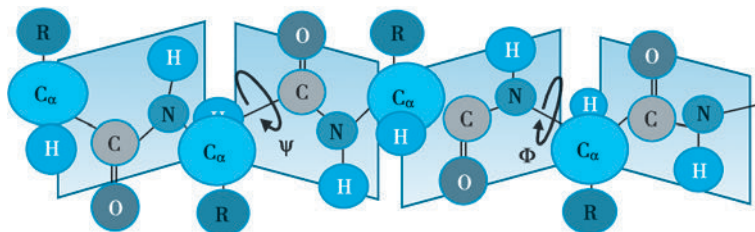
图 1-9 肽键与肽单元
