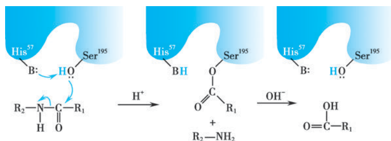
图 2-10 胰凝乳蛋白酶的催化机制
