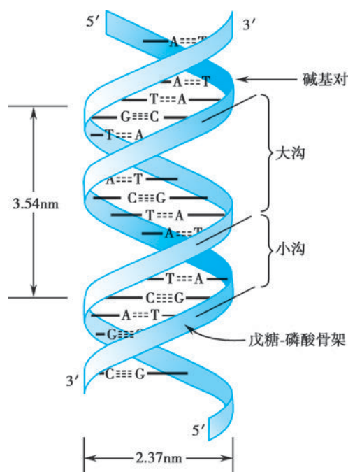
图 3-8 DNA 双螺旋结构的示意图 (侧视图)
