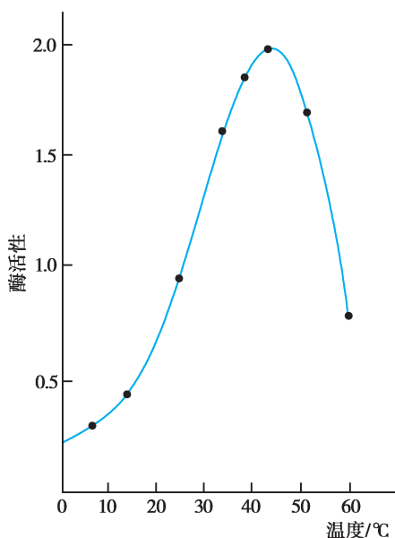
图 2-14 温度对酶促反应速率的影响
