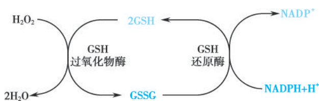
图 1-6 GSH 与 GSSG 间的转换
