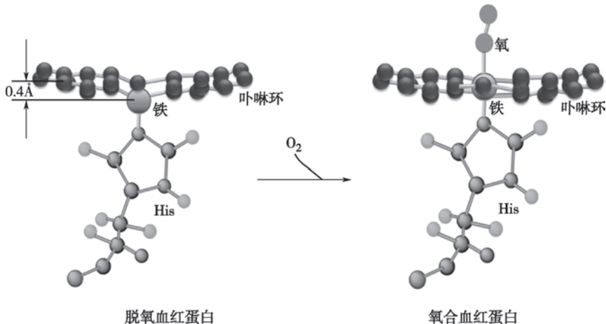
图 1-29 血红素与 O_2 结合
