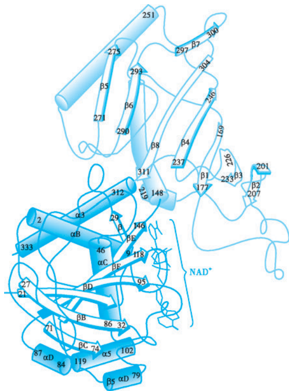
图 1-16 3-磷酸甘油醛脱氢酶亚基的结构示意图
