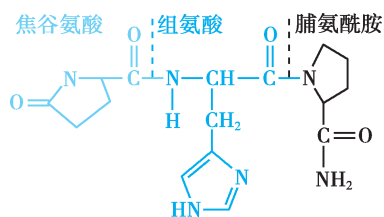
图 1-7 促甲状腺素释放激素的结构
