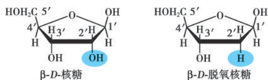
图 3-3 构成核苷酸的核糖和脱氧核糖的化学结构式
