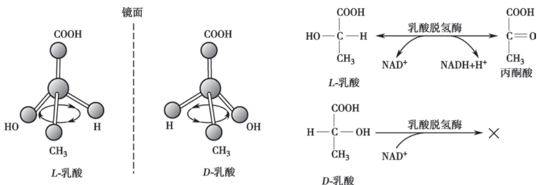
图 2-4 乳酸脱氢酶对乳酸立体异构体的选择性催化
