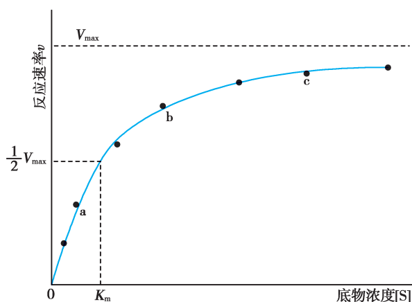
图 2-11 底物浓度对酶促反应速率的影响
