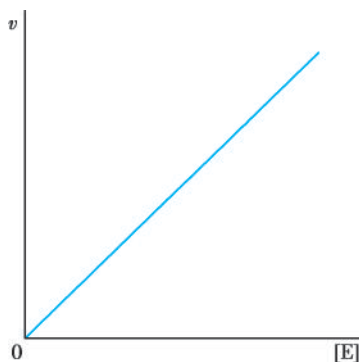
图 2-13 酶浓度对酶促反应速率的影响
