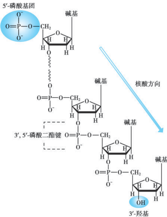
图 3-6 多聚核苷酸的化学结构式
