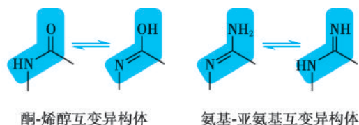
图 3-2 碱基的互变异构式
