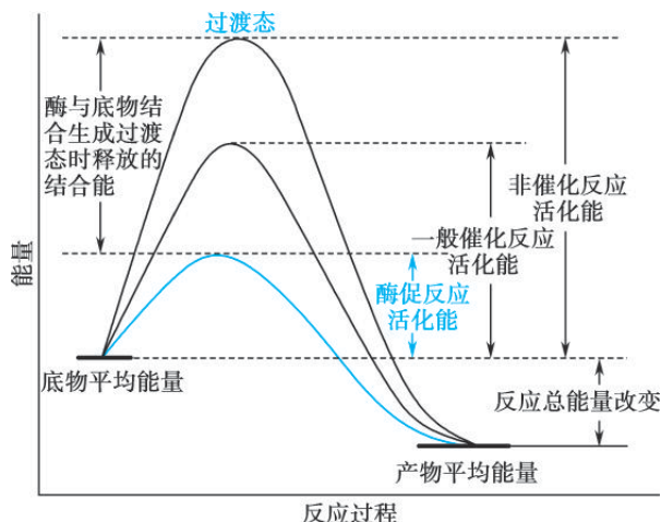
图 2-6 酶促反应活化能的变化
