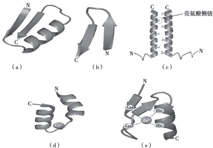
图 1-15 蛋白质超二级结构与模体
