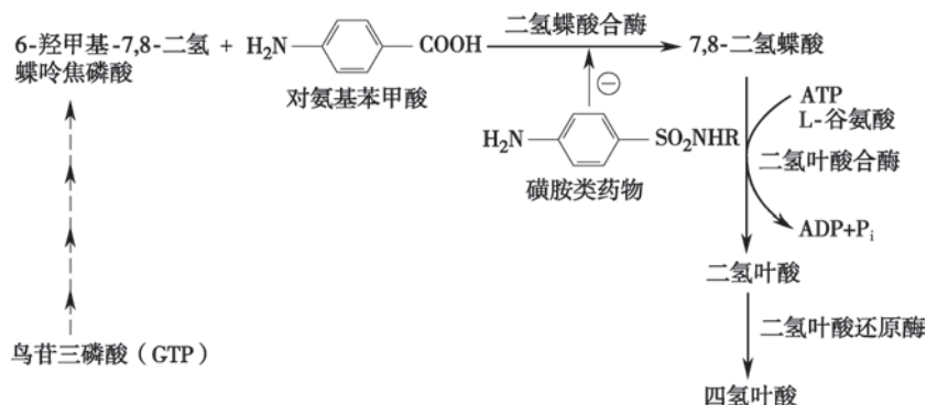
图 2-17 细菌从头合成四氢叶酸的途径和磺胺类药物抑菌的作用机制
