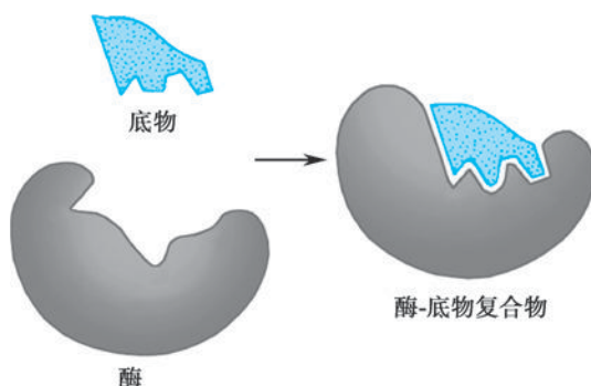
图 2-7 酶与底物结合的诱导契合作用
