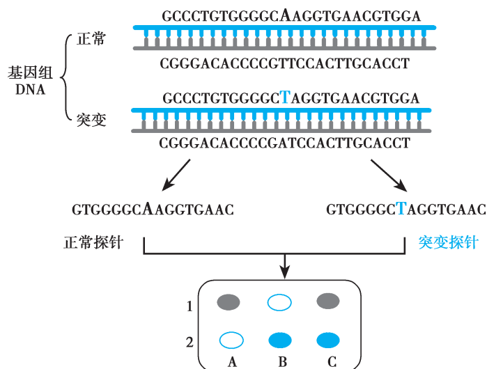
图 24-1 针对β地中海贫血的PCR-ASO分析示意图
