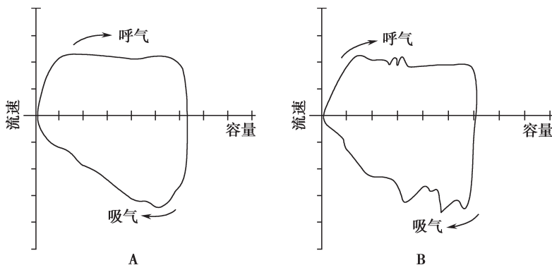
图 4-5 流速 - 容量环
