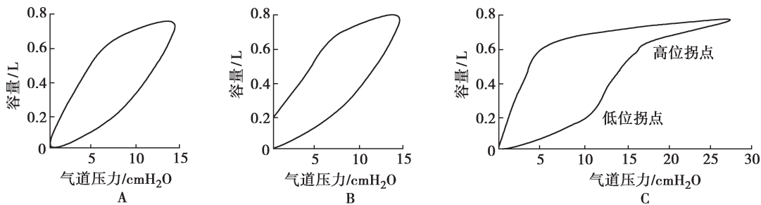
图 4-4 压力 - 容量环
