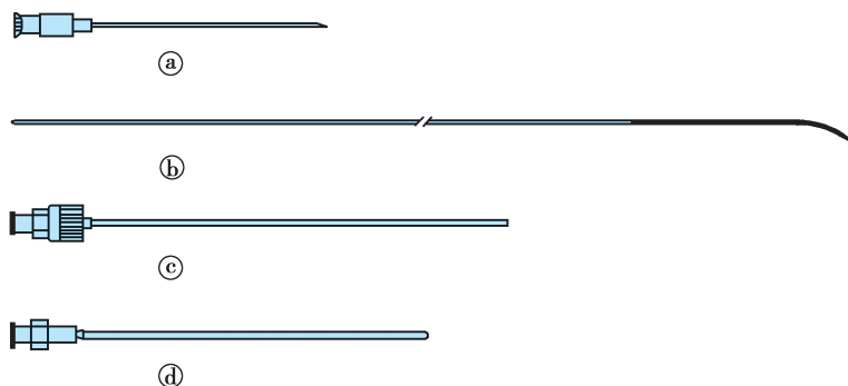
图 12-11 胆道穿刺系统示意图
