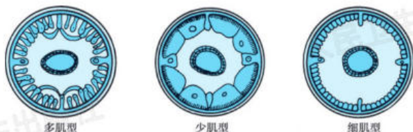
图15-2 线虫的肌型
