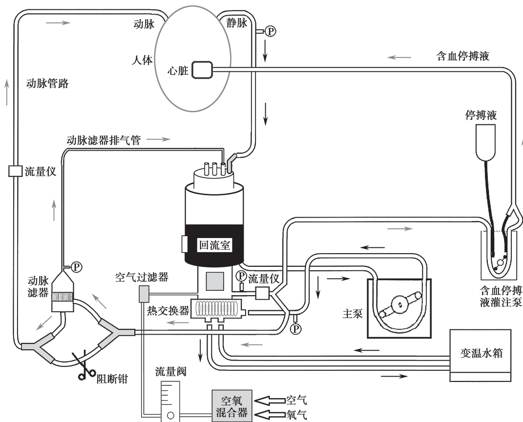
图 13-1 体外循环示意图
