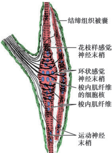
图 7-32 肌梭模式图
