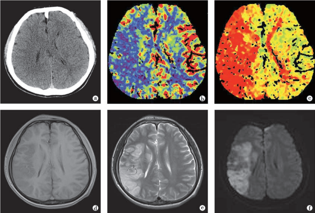
图 2-13 右侧大脑中动脉供血区脑梗死 a. CT 24 小时内难以显示病灶。b. CBF 图像显示右侧额、顶、颞叶,脑室旁脑血流量明显减低。c. 达峰时间 (time to peak, TTP) 图像显示病变区血流灌注达峰时间明显延长。d~f. MRI 右侧额、顶、颞叶,侧脑室旁 T 1 WI 呈低信号 (d), T 2 WI 呈高信号 (e); DWI 呈高信号 (f)。
