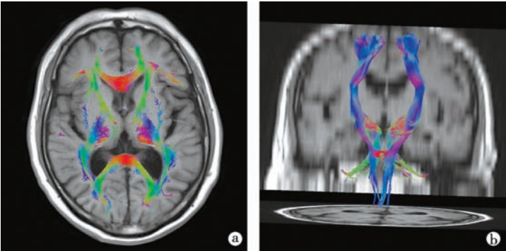
图 2-1 正常脑白质纤维束成像 a. 轴位基底节层面显示伪彩的白质纤维束;b. 冠状面,显示自皮质下向脑干走行的白质纤维束。
