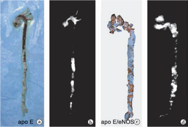
图 1-16 体外对动脉硬化斑块形成中酶的活性成像 a. 未经染色的完整主动脉,白色区域为动脉粥样硬化病灶;b. 用组织蛋白酶-B 激活的分子探针近红外线荧光成像,荧光信号显示形成动脉斑块的位置;c. 主动脉用苏丹染色之后,将血管壁剖开,可见红色区域为动脉粥样硬化病灶;d. 主动脉剖开后的近红外线荧光成像结果,动脉粥样硬化斑块突出于血管壁,组织蛋白酶-B 荧光信号和苏丹染色结果一致。
