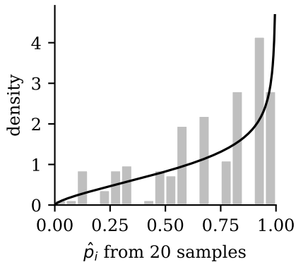
model A: Beta(1.67, 0.72)
