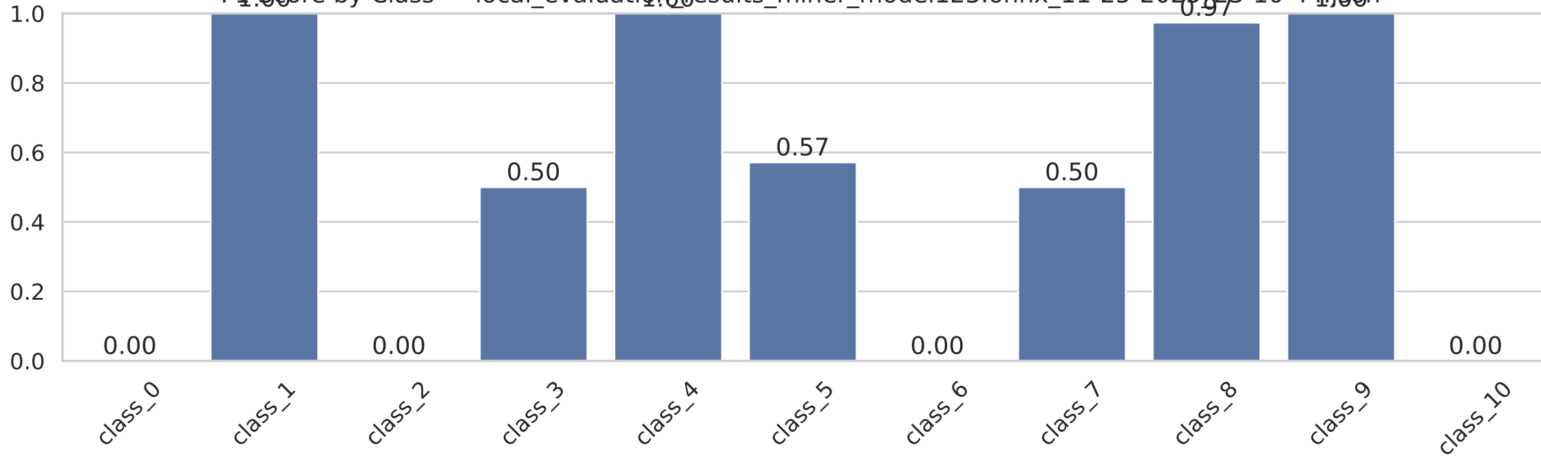
F1 Score by Class — local_evaluation_results_miner_model123.onnx_11-25-2025_23-10-44.json
