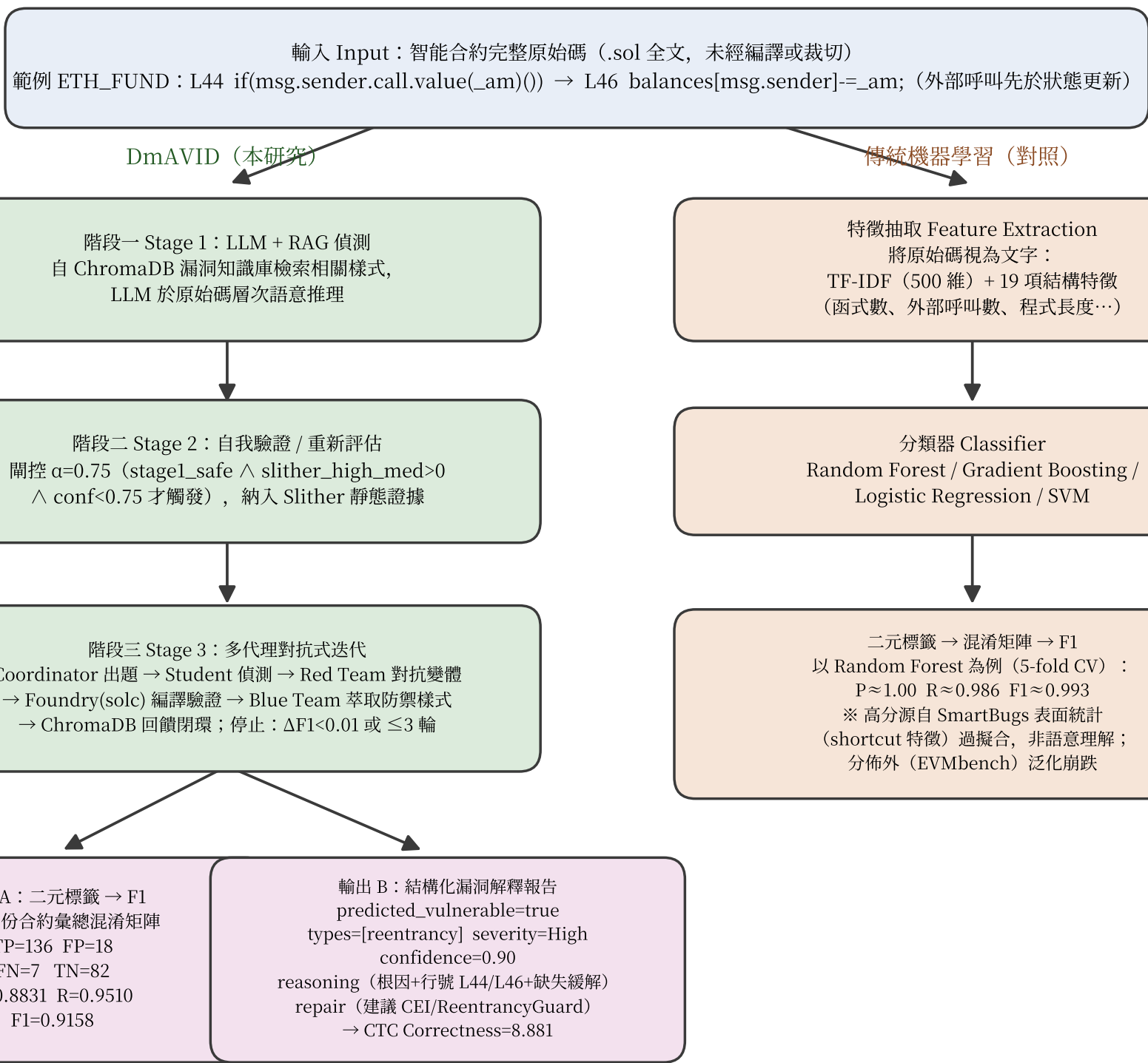
圖 A-1 DmAVID 資訊處理流程：從 .sol 原始碼輸入，至 F1 分數與漏洞解釋報告輸出（並列傳統 ML 對照）
