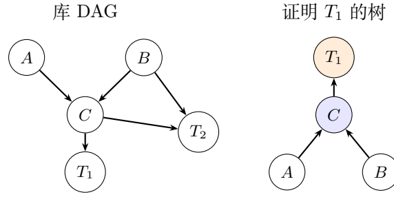
图 3.11: 配图: 纯数学: 引理库 vs 一次证明树
