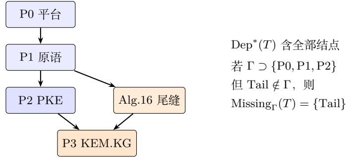
图 3.10: 配图: 工程: KEM.KeyGen 的依赖闭包示意
