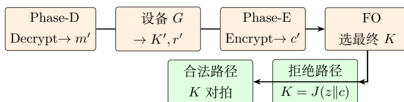
图 7.3: 最小补洞顺序（B 线实际执行）
