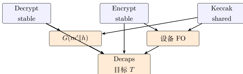
图 7.2: Decaps 实现依赖（写码前从目标反推；仅实现相关）
