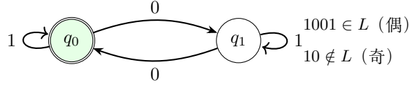
图 3.13: 配图: 纯数学: 偶数个 0 的语言 (附图)
