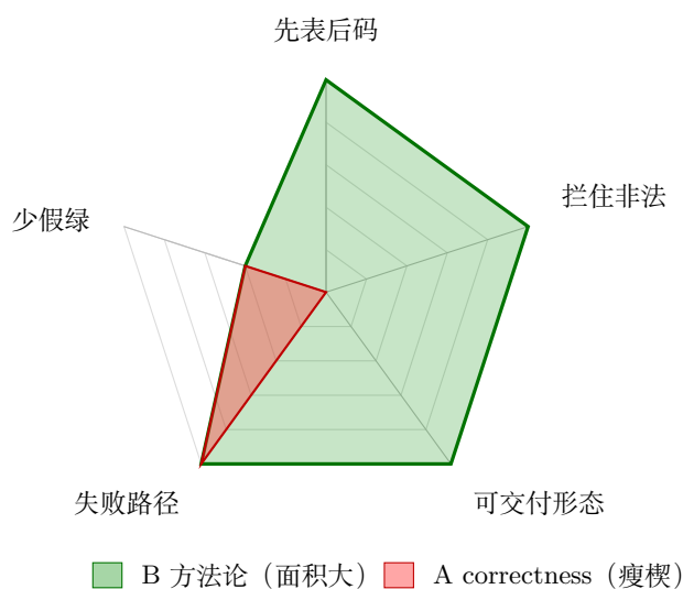
图 7.6: 五指标雷达图: 面积越大越好; B 拉开前四轴, 假绿轴两者一样瘪
