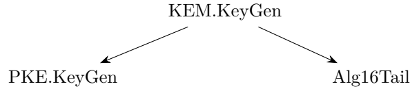
图 3.14: 配图: 工程: KEM.KeyGen 的改写
