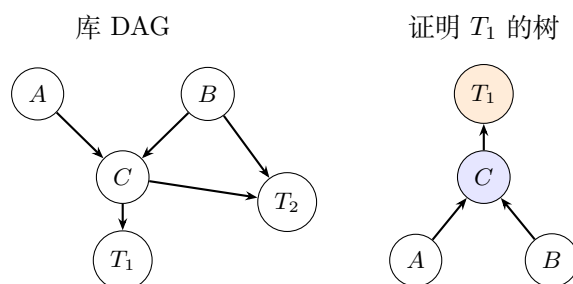
图 3.17: 配图: 纯数学: 引理库 vs 一次证明树
