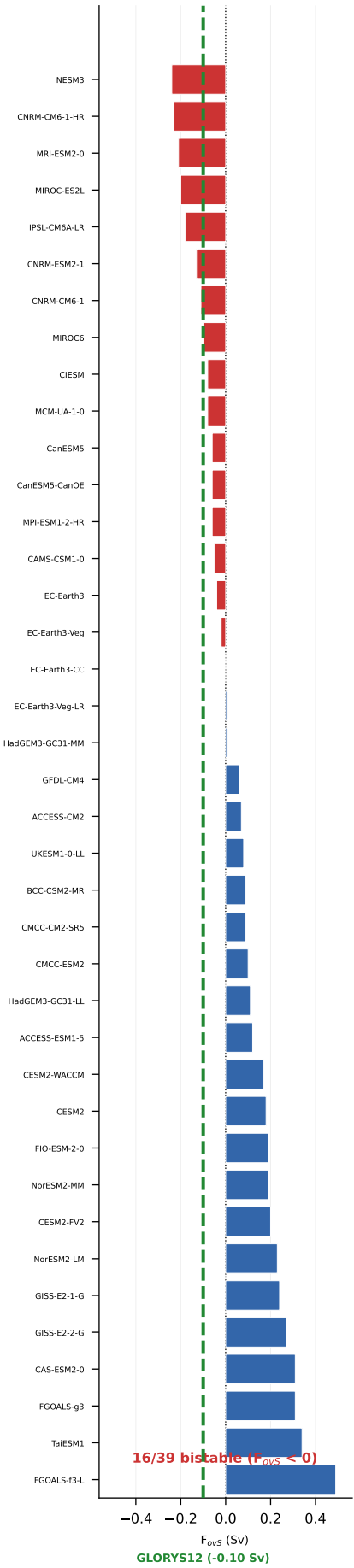
(a) van Westen & Dijkstra 2024 CMIP6, 1994-2020
