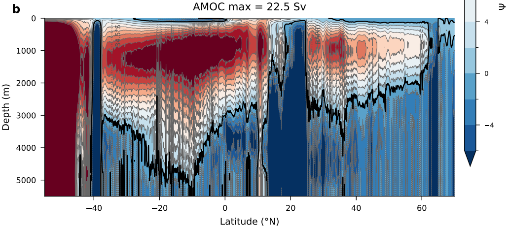
GLORYS12 (2005-2024) AMOC max = 22.5 Sv
