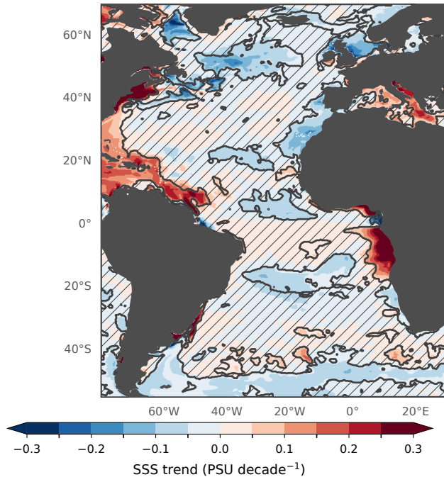
a ORAS5 SSS trend 1993–2025
