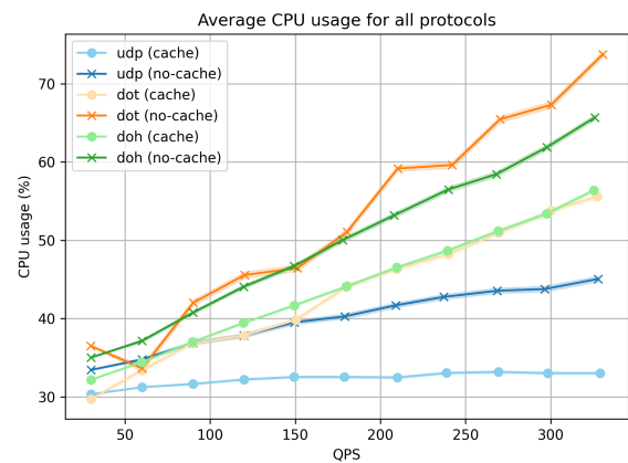
Figure 3.10 – Pourcentage de temps d'activité du CPU pour les différents protocoles avec et sans utilisation du cache
