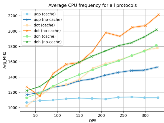
Figure 3.8 – Fréquence moyenne du CPU pour les différents protocoles avec et sans utilisation du cache
