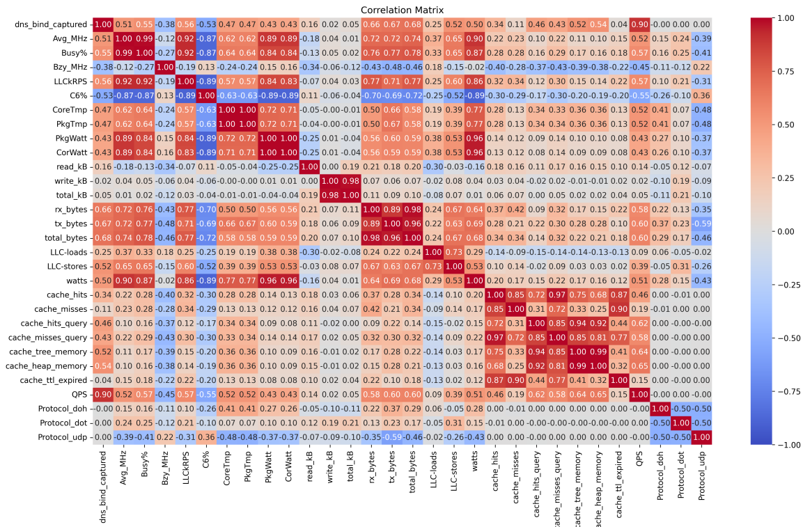
Figure 3.24 – Matrice de corrélation entre les métriques et la consommation énergétique
