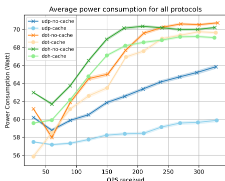
Figure 3.7 – Consommation énergétique moyenne pour UDP, DoT et DoH avec et sans utilisation du cache avec des connexions non persistantes
