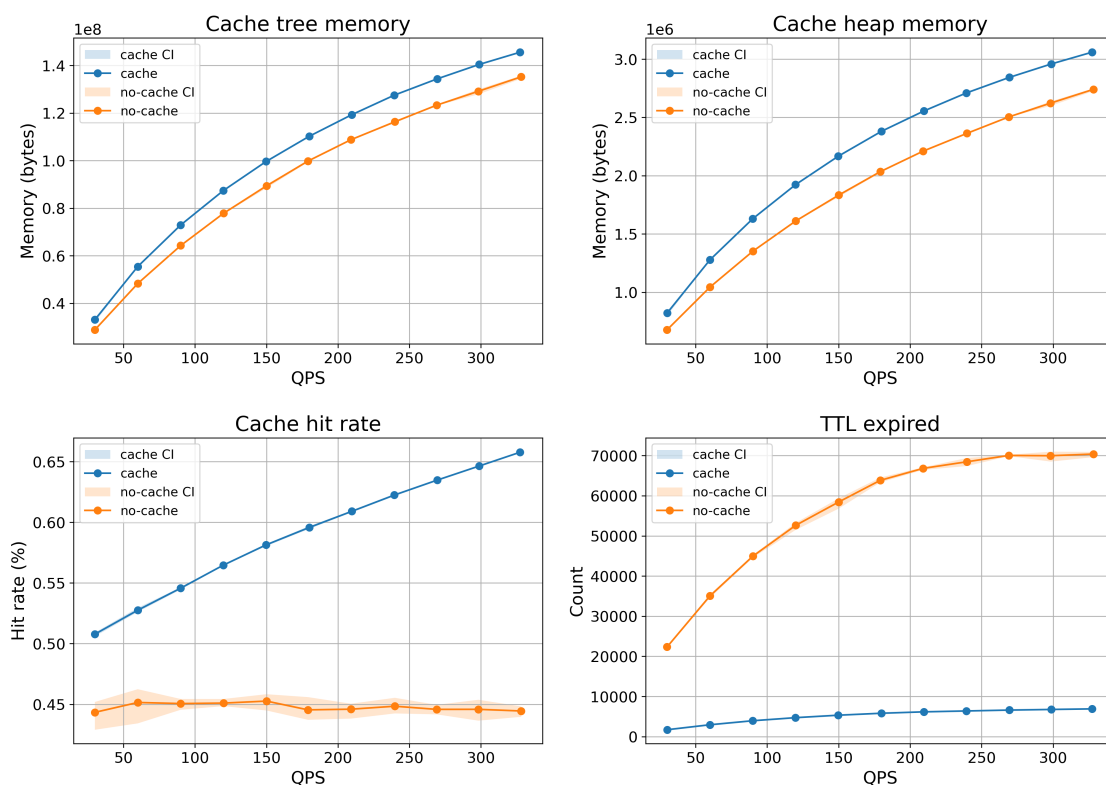
Figure 3.14 – Métriques du cache de Bind9 moyennées pour les différents protocoles avec et sans utilisation du cache
