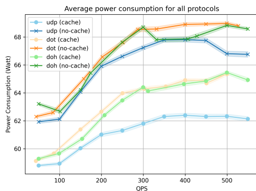
Figure 3.5 – Consommation énergétique moyenne pour UDP, DoT et DoH avec et sans utilisation du cache avec des connexions persistantes
