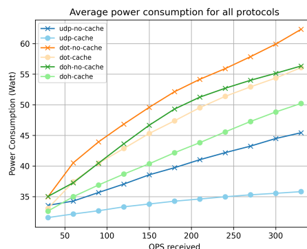
Figure 3.8 – Consommation énergétique moyenne pour UDP, DoT et DoH avec et sans utilisation du cache avec des connexions non persistantes, sans la surcharge lié à l'enregistrement des métriques au niveau du DNS
