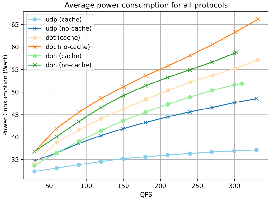
Figure 3.9 – Consommation énergétique moyenne pour UDP, DoT et DoH avec et sans utilisation du cache avec des connexions non persistantes, sans la surcharge lié à l'outil de mesure rndc
