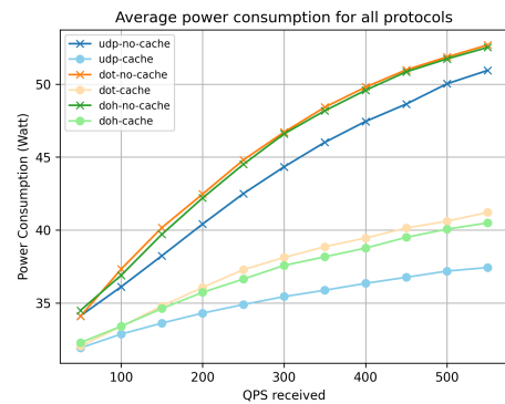
Figure 3.6 – Consommation énergétique moyenne pour UDP, DoT et DoH avec et sans utilisation du cache avec des connexions non persistantes, sans la surcharge liée à l'enregistrement des métriques au niveau du DNS
