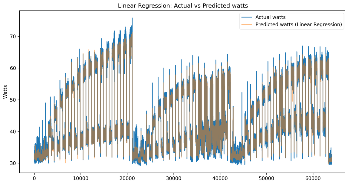
Figure 3.15 – Estimation par régression linéaire et consommation énergétique réelle
