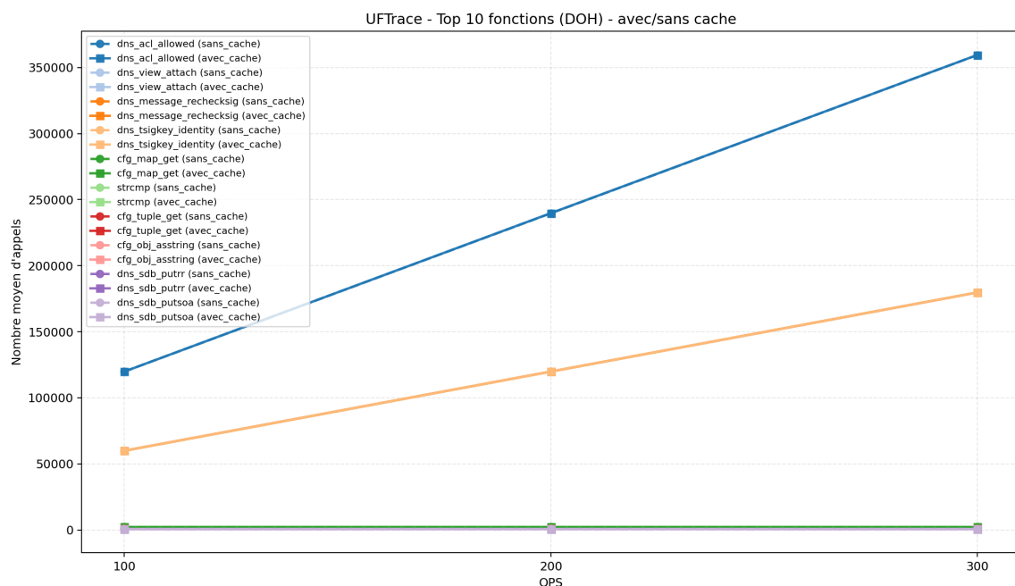
Figure 3.14 – Nombre d'appels des 10 fonctions les plus appelées de Bind9 en fonction du QPS pour DoH avec utilisation du cache
