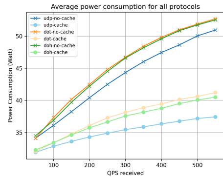
Figure 3.6 – Consommation énergétique moyenne pour UDP, DoT et DoH avec et sans utilisation du cache avec des connexions non persistantes, sans la surcharge liée à l'enregistrement des métriques au niveau du DNS
