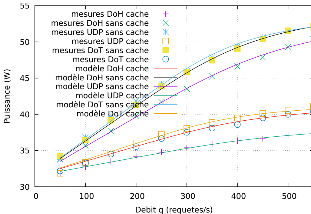
Figure 3.25 – Comparaison modèle-mesures dans la plage expérimentale.
