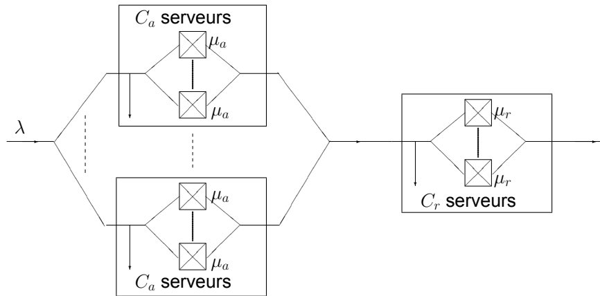
Figure 3.24 – Modèle approché de bind9
