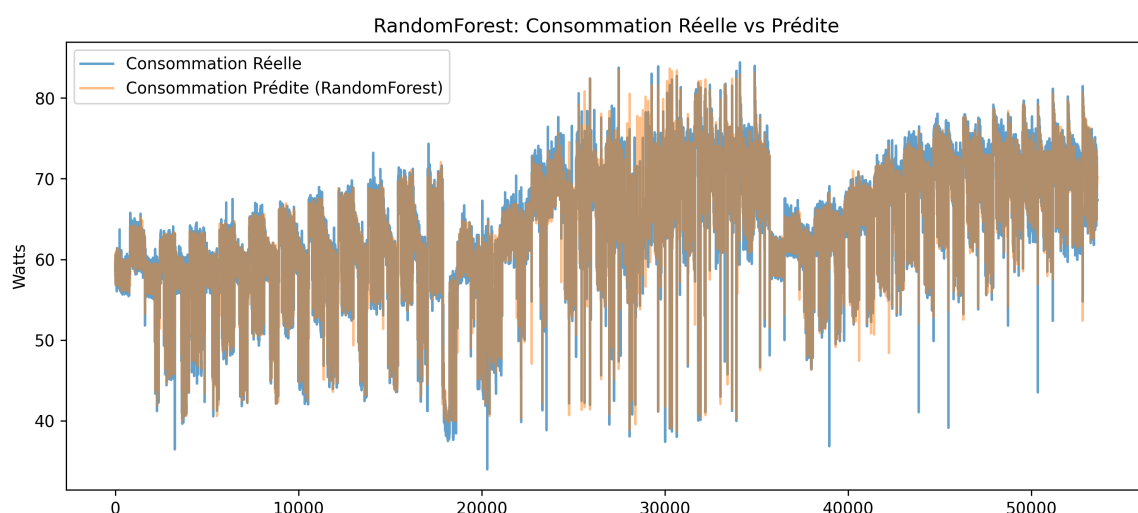
Figure 3.22 – Estimation par RandomForest et consommation énergétique réelle, montrant une bonne prédiction de la puissance consommée.
