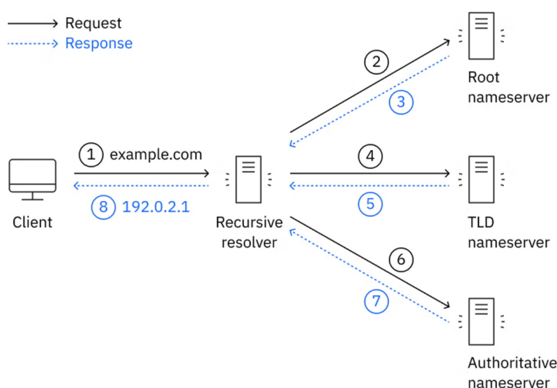
Figure 2.1 – Exemple simplifié d'une résolution DNS récursive.
