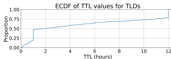
Figure 3.16 – Distribution des TTL pour les TLD
