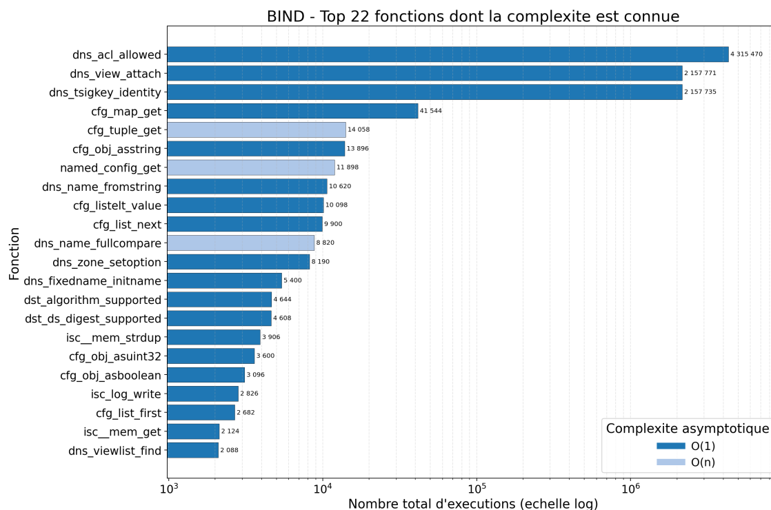
Figure 3.21 – Nombre d'appels des 22 fonctions les plus appelées de Bind9 avec leur complexité algorithmique statique
