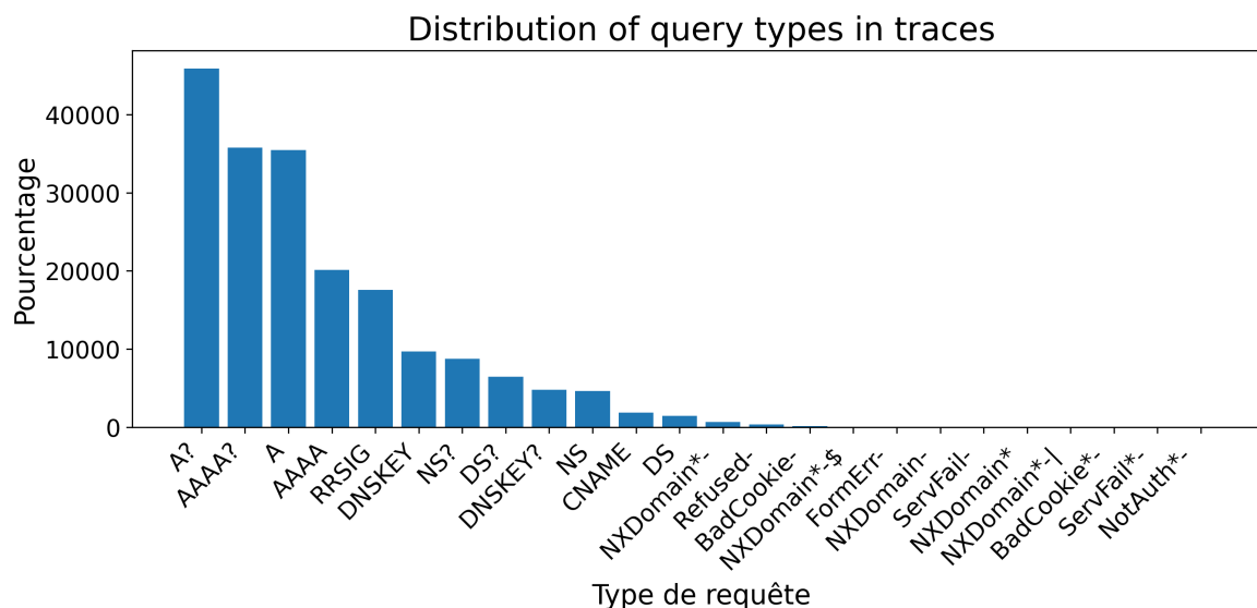
Figure 3.14 – Distribution des types de requêtes pour les résolutions récursives
