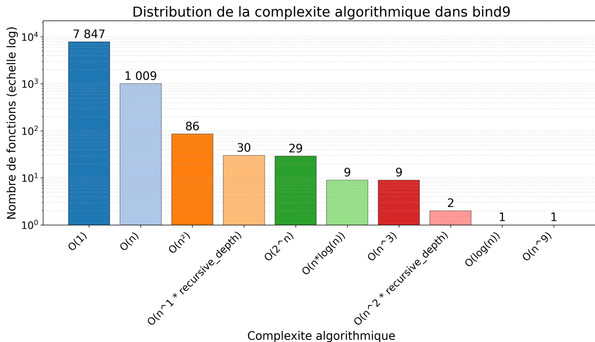
Figure 3.17 – Graphiques de l’analyse de la complexité algorithmique statique de Bind9
