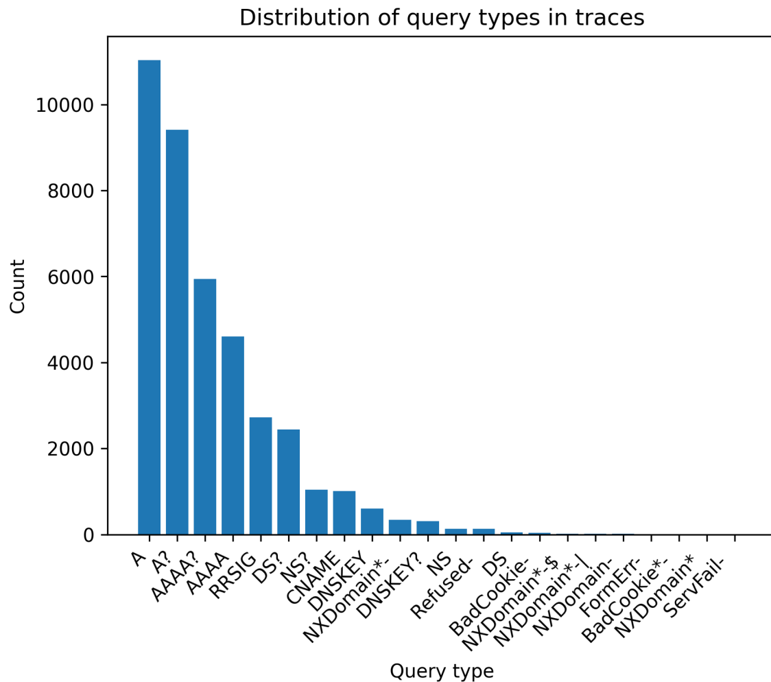
Figure 3.5 – Distribution des types de requêtes pour les résolutions récursives
