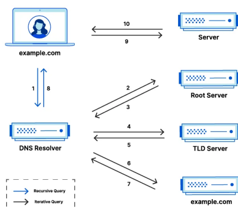
Figure 3.1 – Exemple simplifié d'une résolution DNS récursive.
