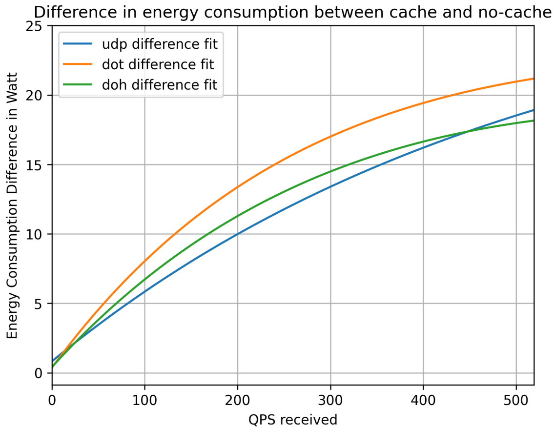
Figure 3.4 – Différence de consommation entre les résolutions avec et sans cache
