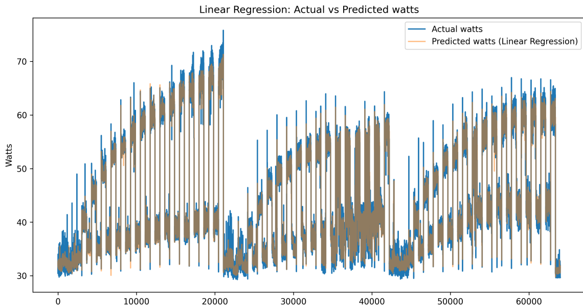
Figure 3.6 – Estimation par régression linéaire et consommation énergétique réelle
