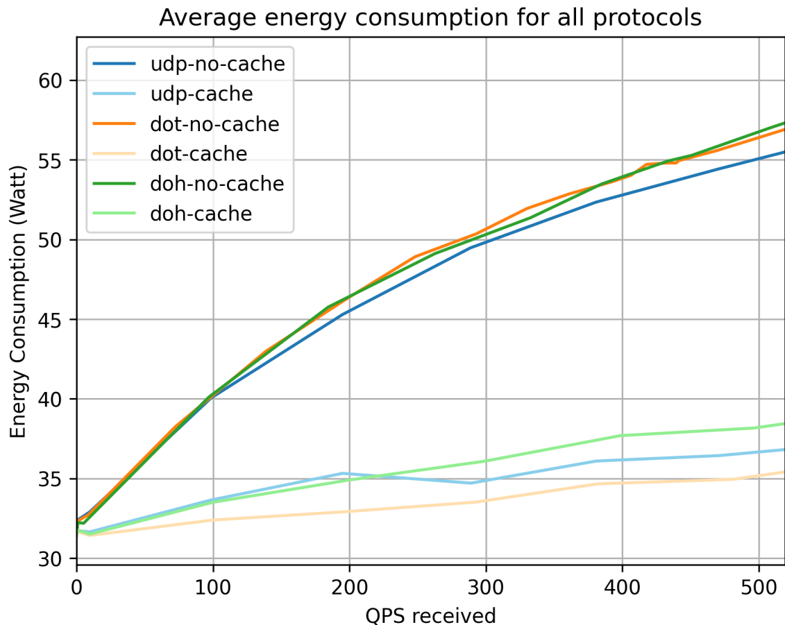
Figure 3.2 – Consommation énergétique moyenne pour UDP, DoT et DoH avec et sans utilisation du cache
