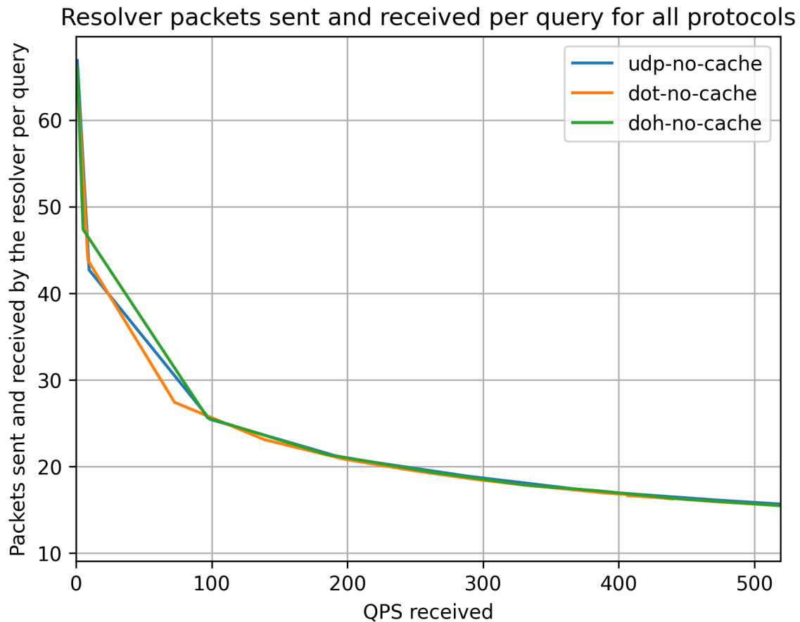
Figure 3.3 – Nombre de requêtes envoyées et reçues par le résolveur pour une résolution en fonction du QPS
