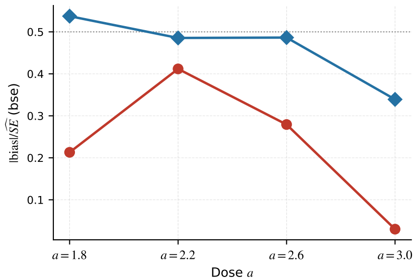
Kernel DR (DRKPV)
