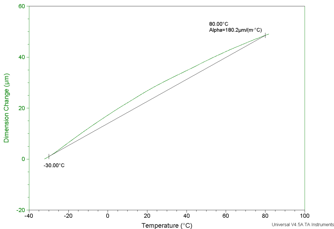
样品 A2170021539101003 厚度方向线性热膨胀系数测试曲线
