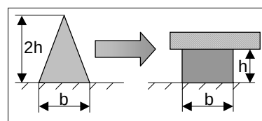
图 2: 推荐的胶条形状
