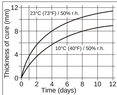
图表 1: Sikaflex®-265 的固化速度
