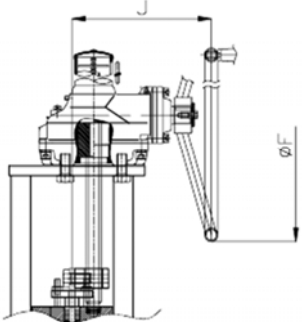
2) 6~10" Bevel Gear
