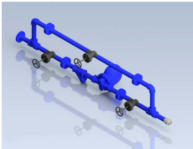
SISTEMA DE TRAMPEO CON BY-PASS
