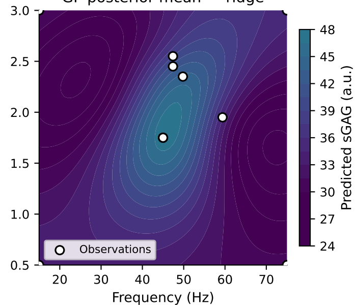
GP posterior mean — ridge
