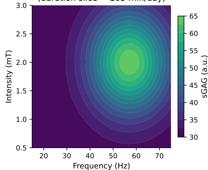
GP posterior mean — unimodal
