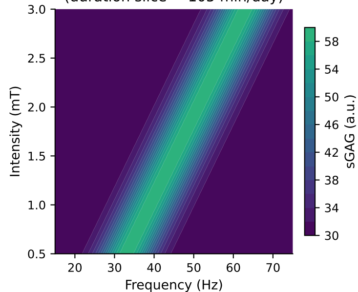
GP posterior mean — ridge
