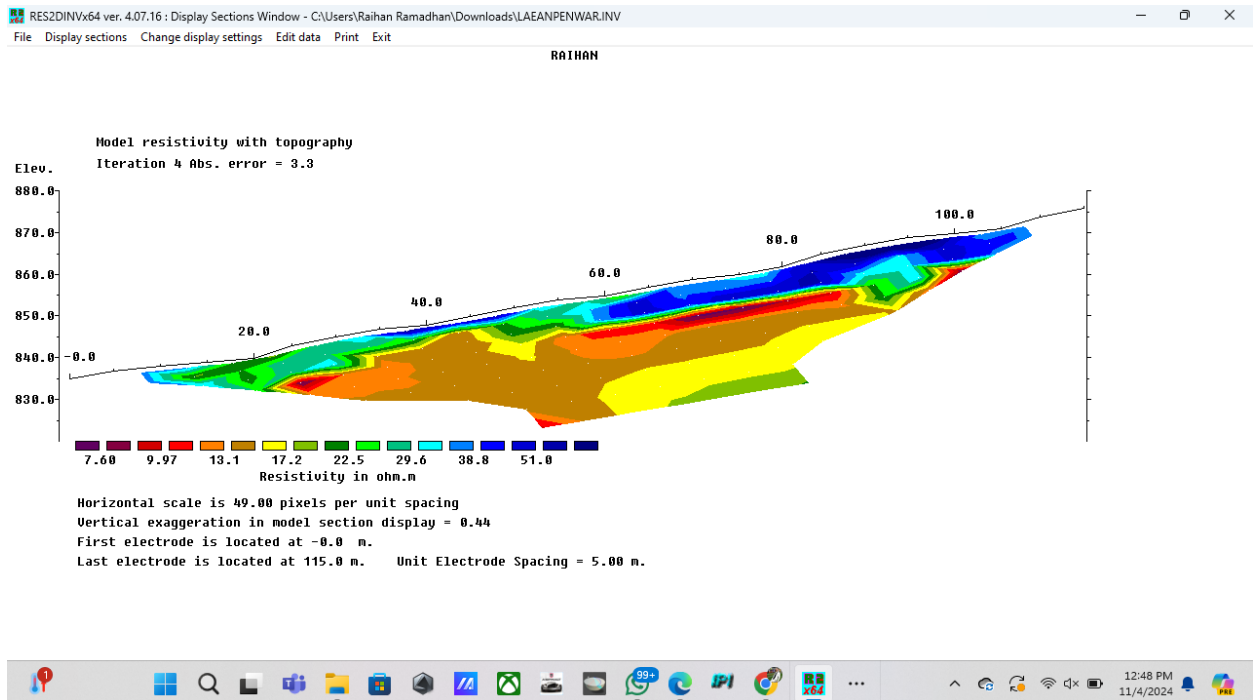
Gambar 2. Penampang resistivity dengan topografi
