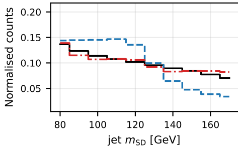
50% QCD mis-id
