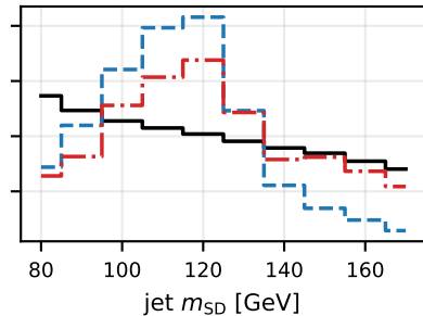
1% QCD mis-id
