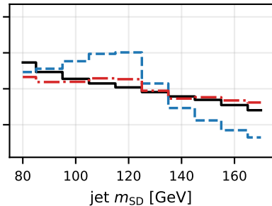
10% QCD mis-id
