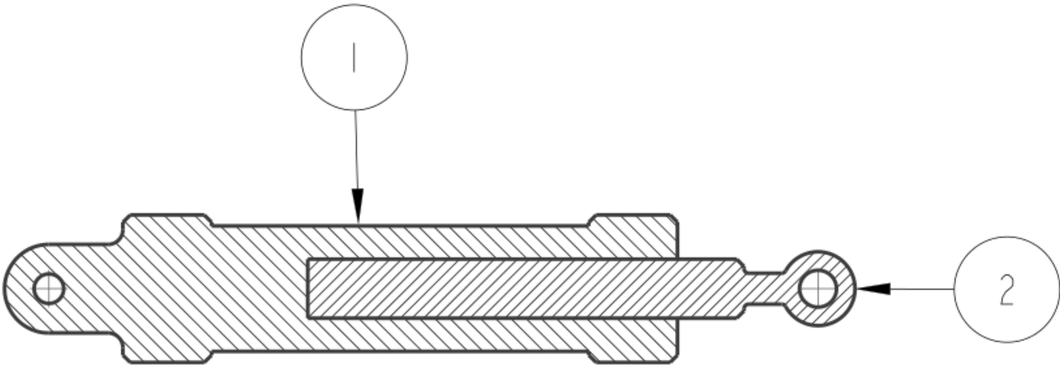
SECTION A-A
