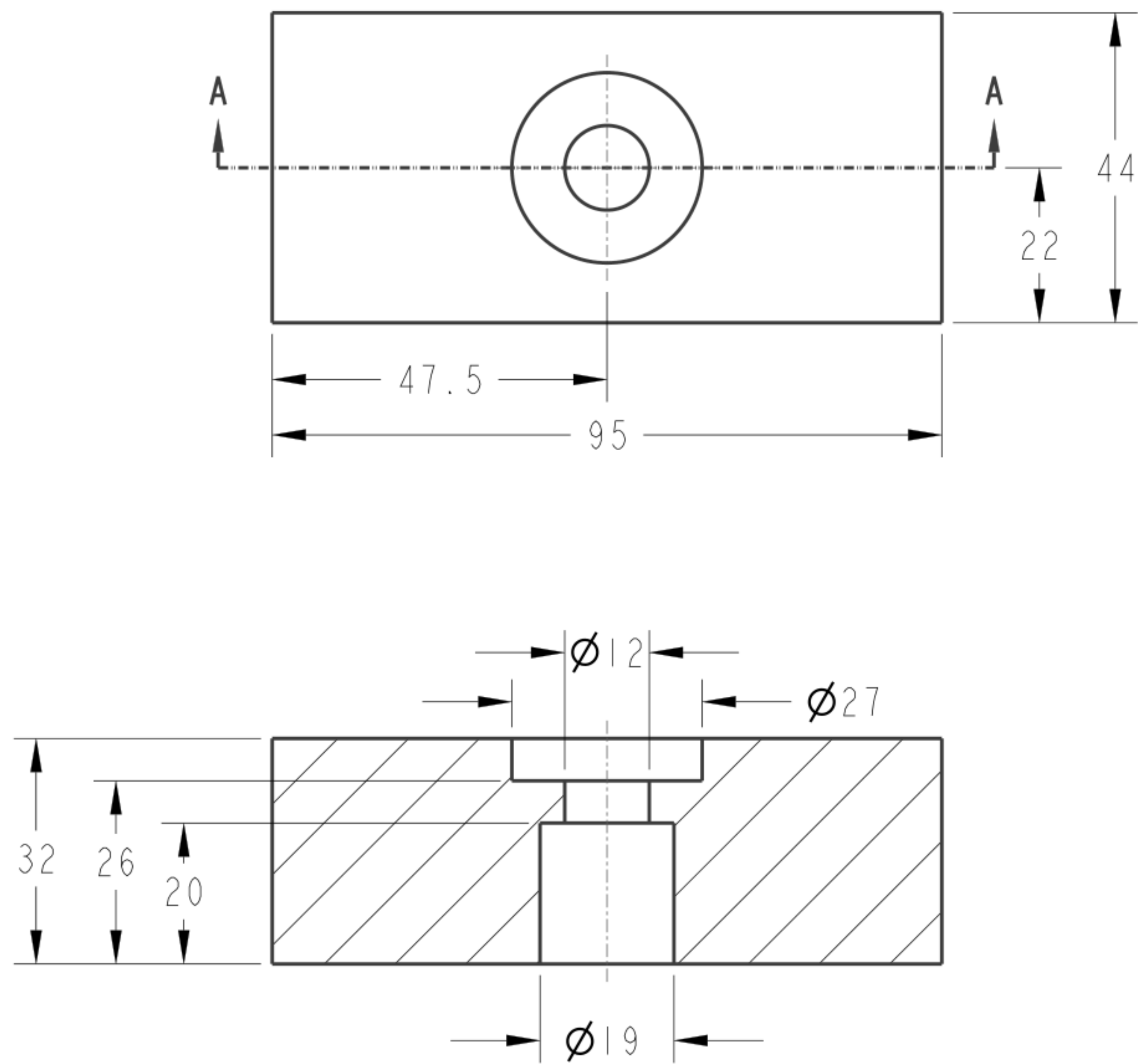
SECTION A-A
