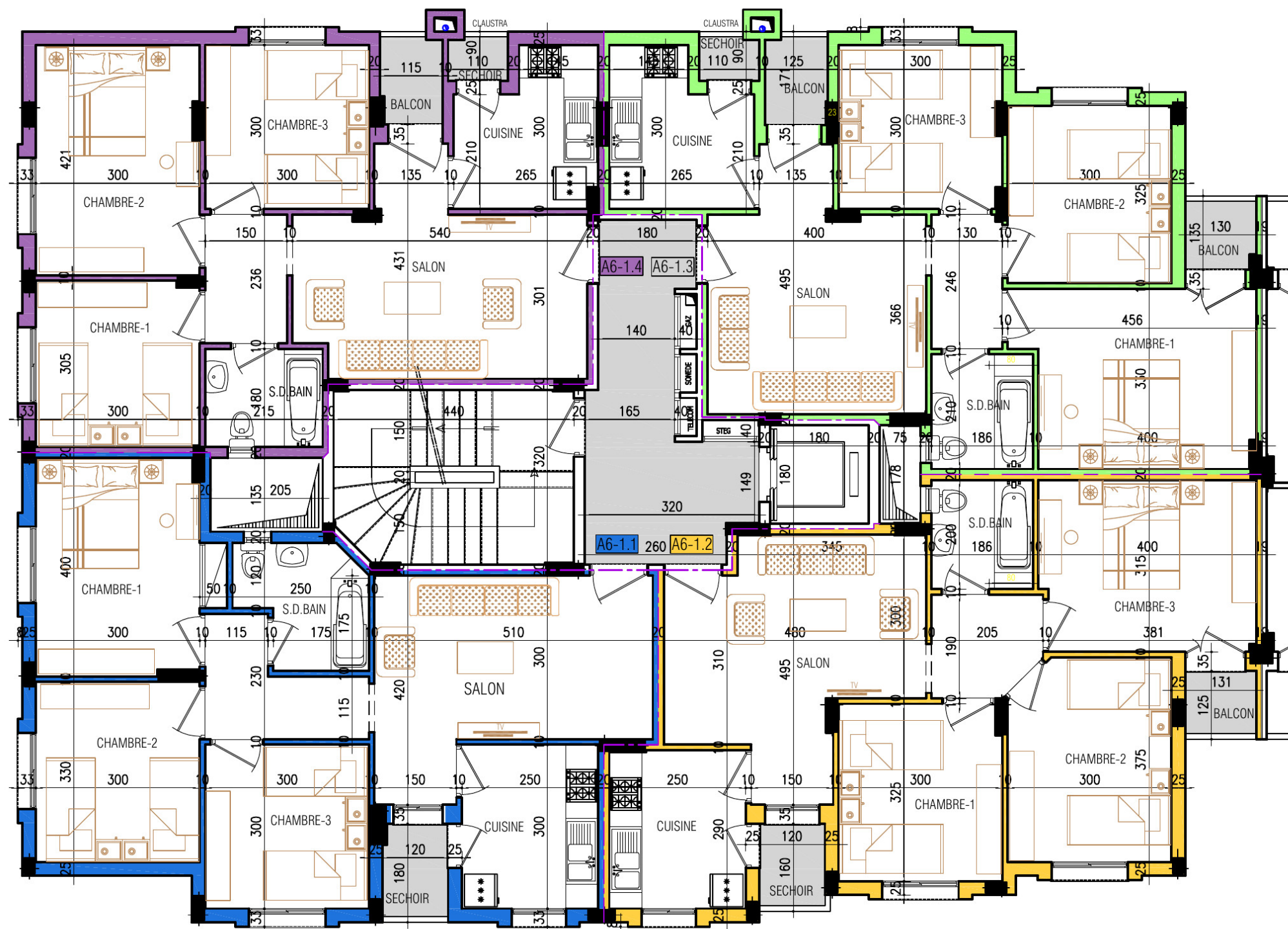
PLAN 1er ETAGE
