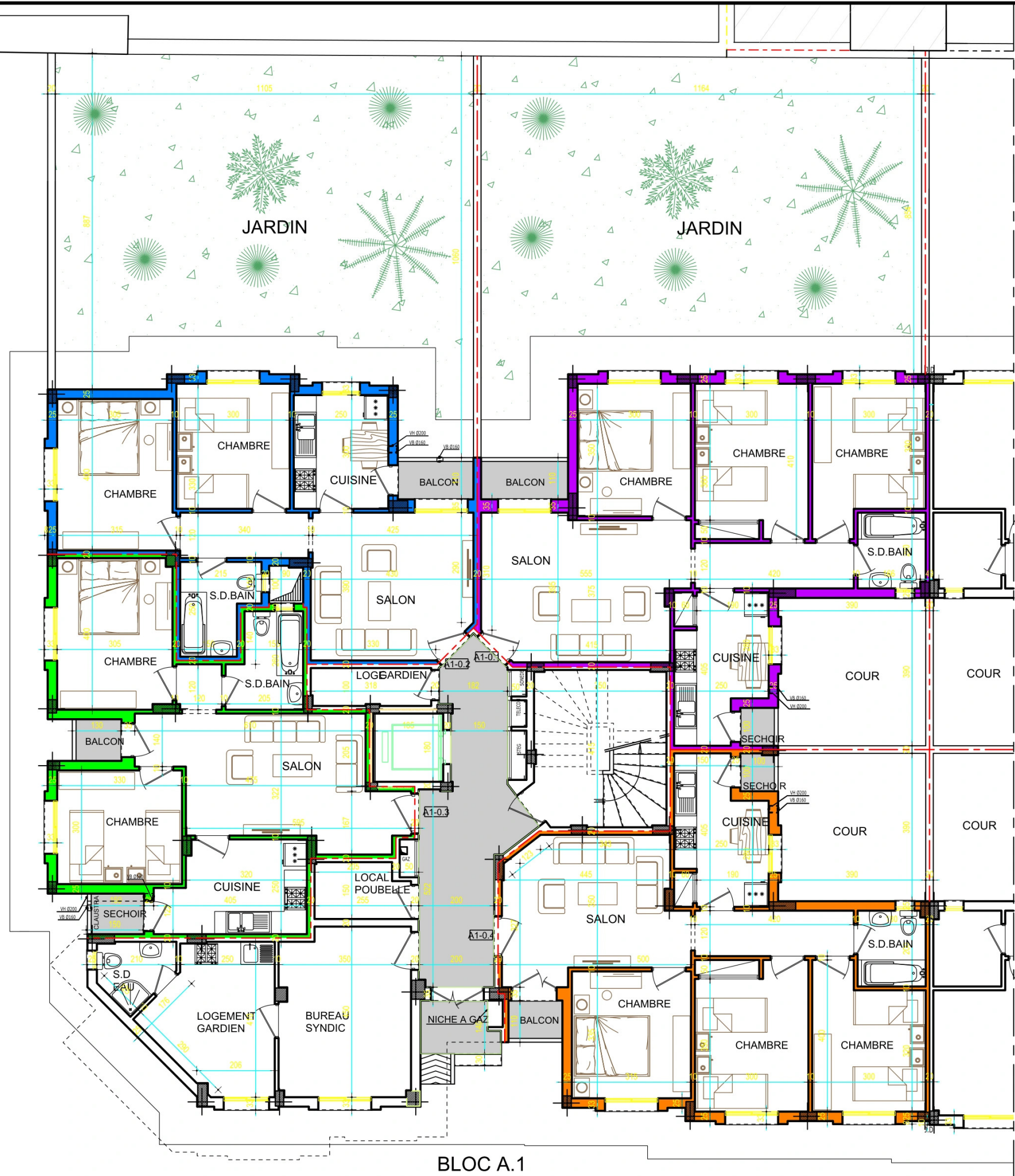
PLAN REZ-DE-CHAUSSEE
